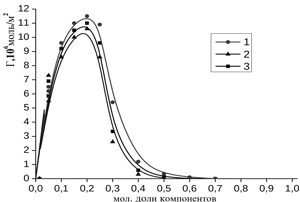
Рисунок 7 – Изотерма адсорбции компонентов в системе ацетон – диоксан 1.4 – вода при 293 К. 1 – адсорбция ацетона в системе вода – ацетон ; 2 – адсорбция диоксана 1.4 в системе вода – диоксан 1.4 ; 3 – суммарная адсорбция ацетона и диоксана 1.4 в тройной системе при изменении составов по сечениям X_{\text{ац-н.}} : X_{\text{диок.}} = 1:1
