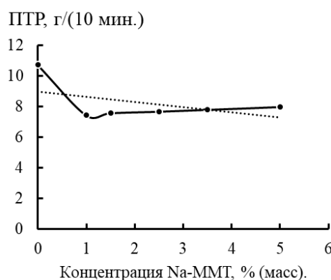
Рисунок 1 – Концентрационная зависимость предела текучести расплава ПБТ и композиции ПБТ + Na-MMT 1%; ПБТ + Na-MMT 1,5%; ПБТ + Na-MMT 2,5 %; ПБТ + Na-MMT 3,5 %; ПБТ + Na-MMT 5%.
