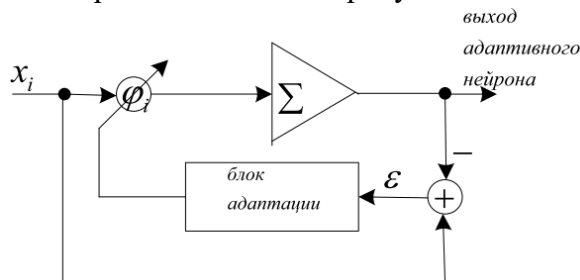
Рисунок 2 – Схема адаптивного нейрона линейного порядка, используемого в первом слое модифицированной нейро-нечеткой продукционной сети Anfis
