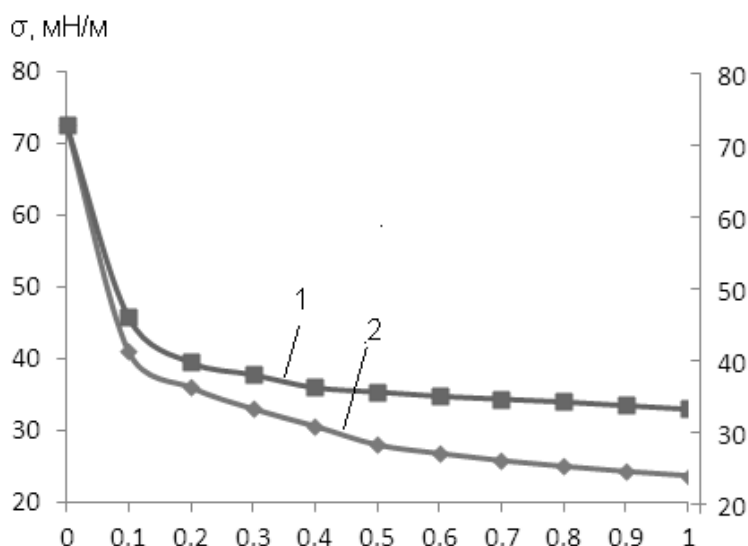
Рисунок 5 – Зависимость поверхностного натяжения от молярных долей второго компонента двойной системы: 1- вода – диоксан 1.4; 2- вода – ацетон при 293 К.
