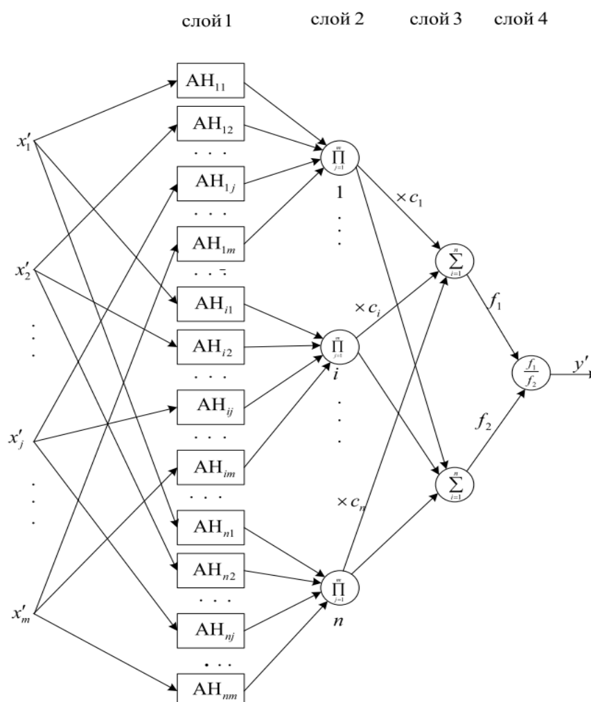
Рисунок 3 – Структурная схема модифицированной нейро-нечеткой продукционной сети Anfis, использующей алгоритм Ванга-Менделя
