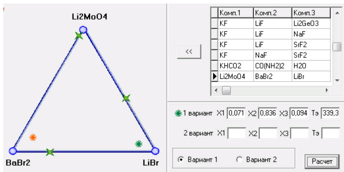
Рисунок 5 – Вычисление температуры и состава эвтектики секущего треугольника
