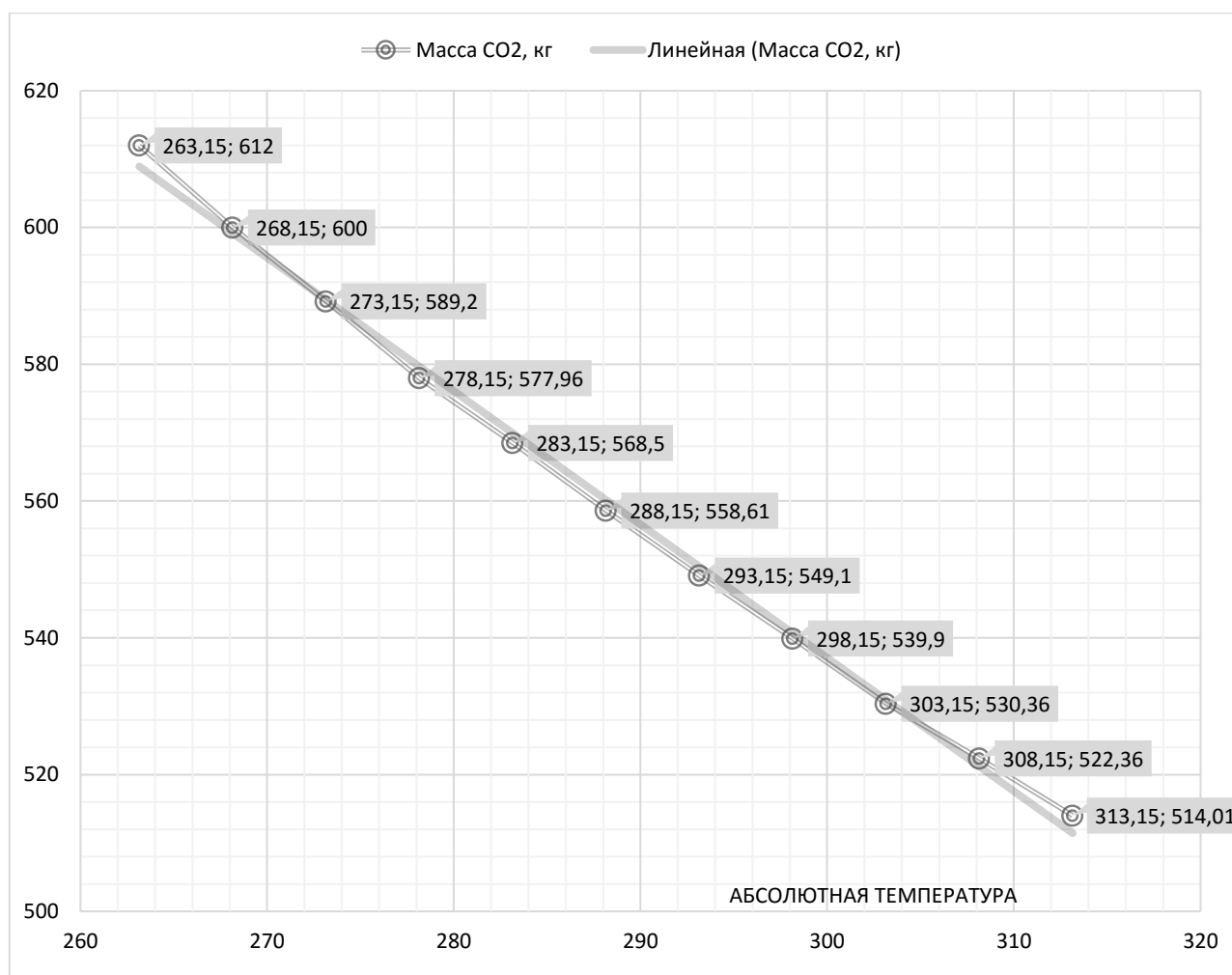
Рисунок 1в – Столбчатая диаграмма зависимости содержания массы углекислого газа CO 2 в слое воздуха высотой 100 м над пашней площадью в 1га от температуры окружающей среды
