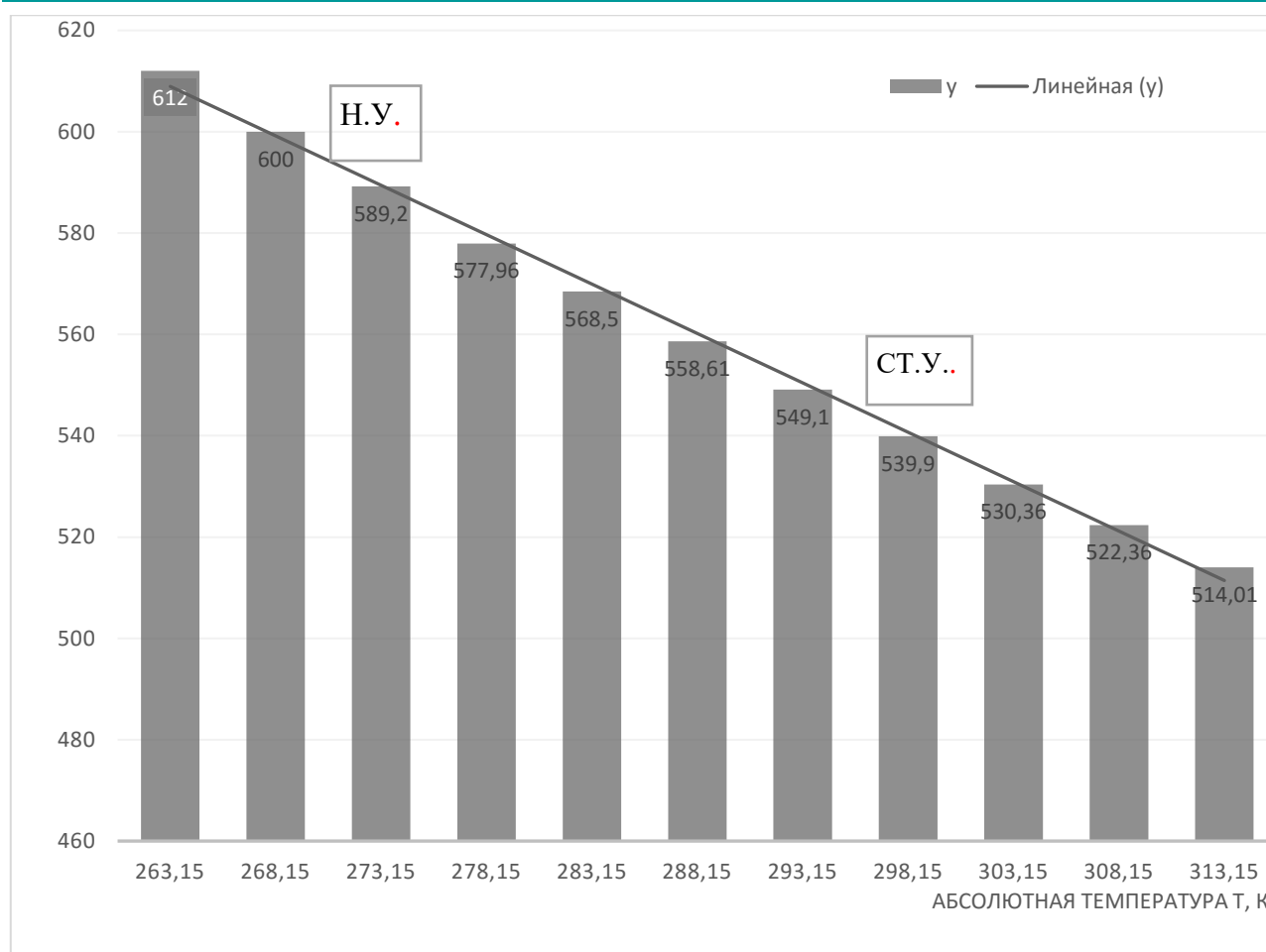
Рисунок 1а – Столбчатая диаграмма зависимости содержания массы углекислого газа \text{CO}_2 в слое воздуха высотой 100 м над пашней площадью в 1га от температуры окружающей среды
