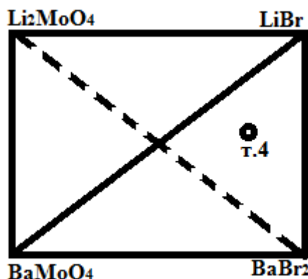
Рисунок 3 – Квадрат составов системы \text{Li}^+, \text{Ba}^{2+} || \text{MoO}_4^{2-}, \text{Br}^-
