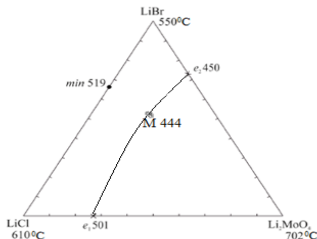
Рисунок 2 – Фазовый комплекс трехкомпонентной системы \text{LiCl-LiBr-Li}_2\text{MoO}_4
