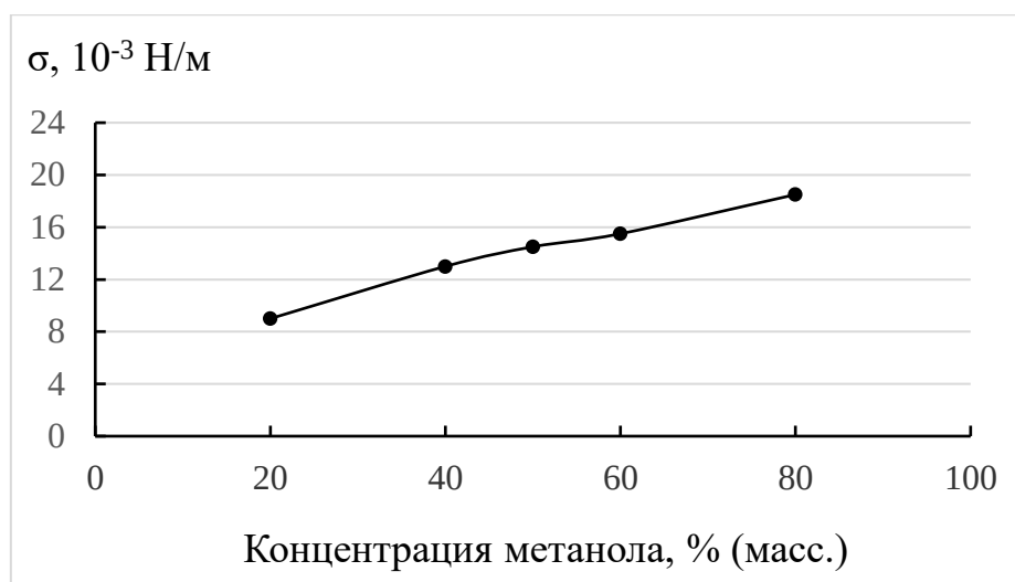
Рисунок 8 – Поверхностное натяжение в зависимости от концентрации метилового спирта
