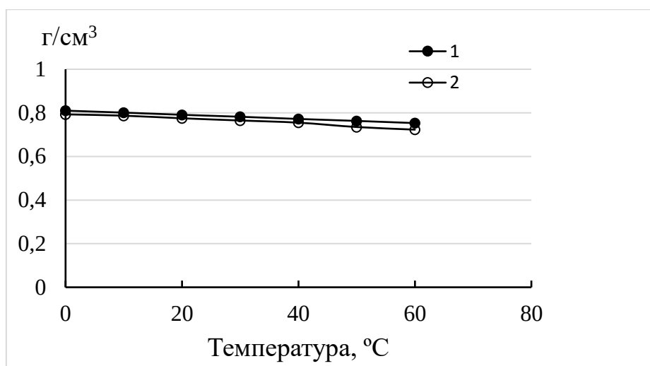
Рисунок 3 – Плотность метилового спирта в зависимости от температуры
