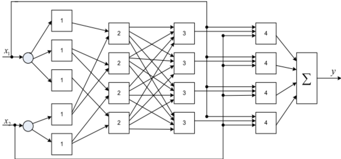
Рисунок 1 – Нейро-нечеткая Anfis, использующая алгоритм Сугено-Такаги нулевого порядка
