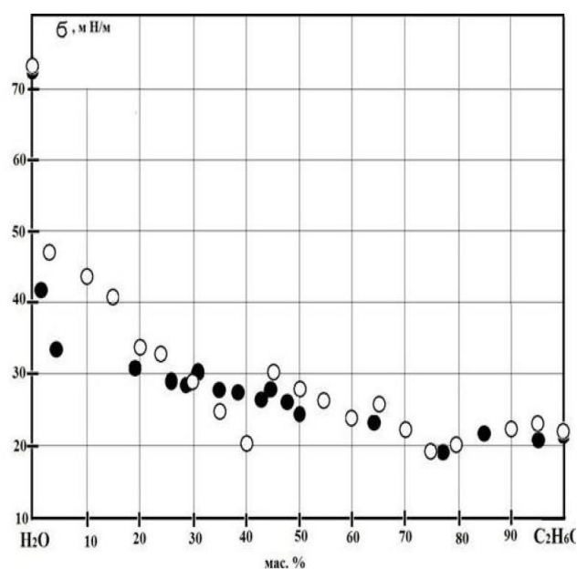
Рисунок 6 – Концентрационная зависимость изотермы поверхностного натяжения водного раствора этилового спирта, при 22 °С:
