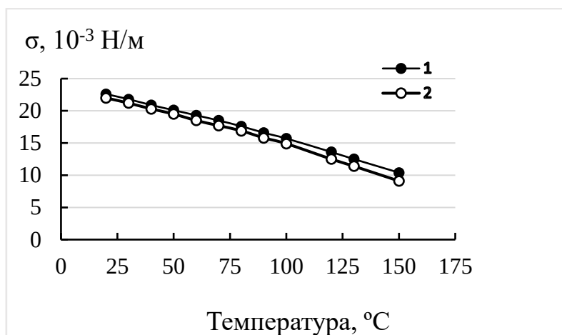
Рисунок 7 – Поверхностное натяжение метилового спирта в зависимости от температуры
