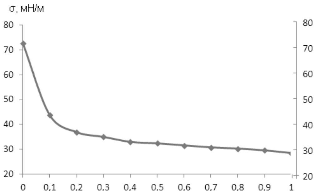
Рисунок 6 – Изотерма поверхностного натяжения системы вода – ацетон - диоксан 1.4 при 293 К.
