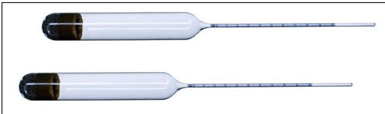
Рисунок 1– Ареометр. Предназначен для измерения объемной концентрации спирта в водных растворах. Ареометры изготовлены в соответствии с ГОСТ 18481-81.
