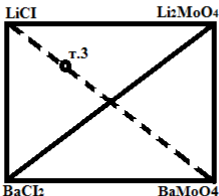
Рисунок 2– Квадрат составов системы Li^+, Ba^{2+} || MoO_4^{2-}, Cl^-
