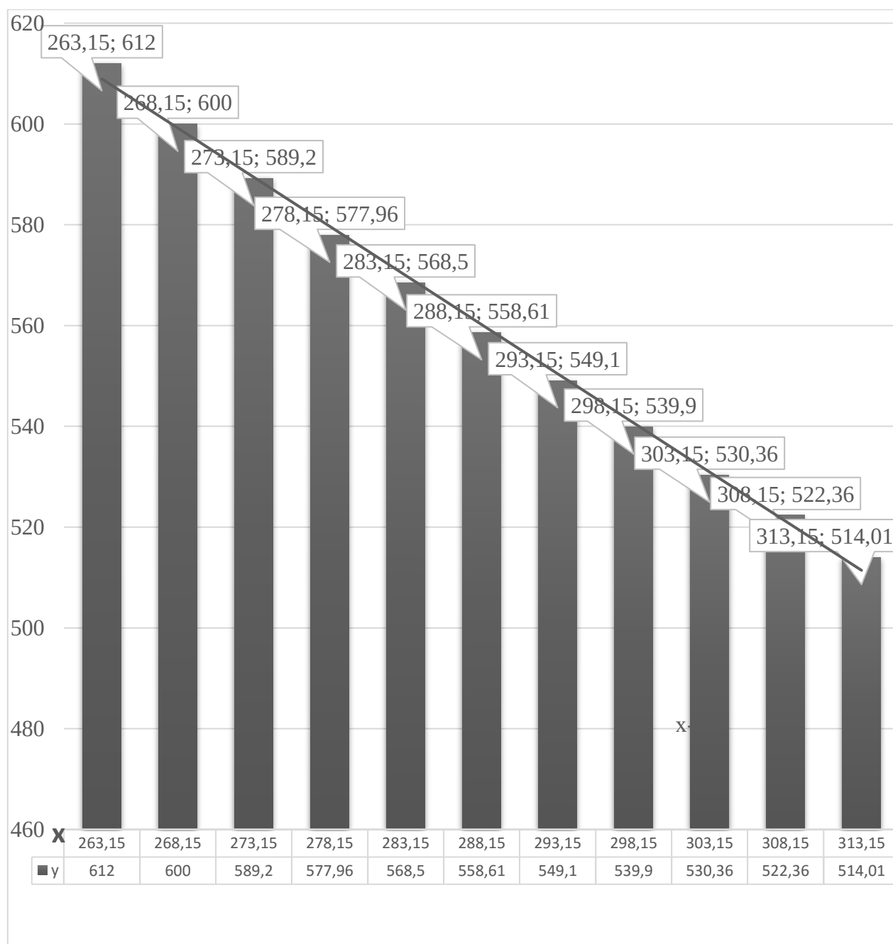
Рисунок 1б – Столбчатая диаграмма зависимости содержания массы углекислого газа CO 2 в слое воздуха высотой 100 м над пашней площадью в 1га от температуры окружающей среды.
