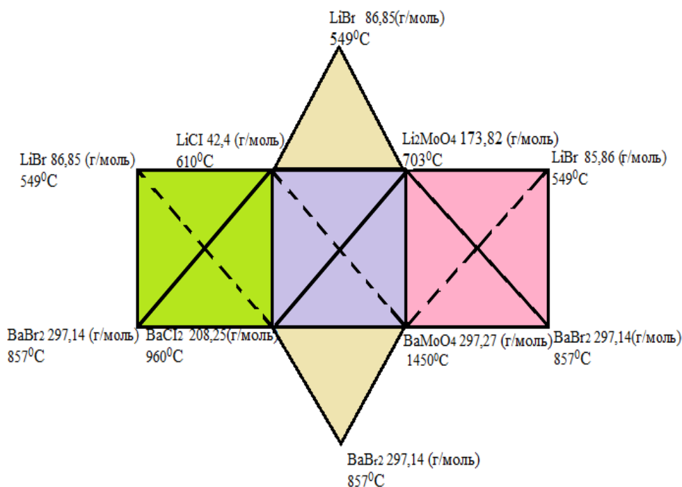
Рисунок 1 – Призма и развертка состава четырехкомпонентной взаимной системы \text{Li, Ba} || \text{Br, Cl, MoO}_4
