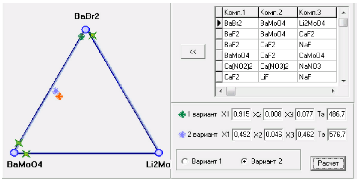
Рисунок 6 – Вычисление температуры и состава эвтектики секущего треугольника
