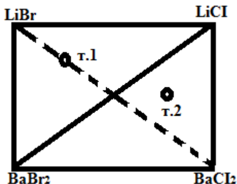
Рисунок 1 – Квадрат составов системы Li^+, Ba^{2+} || Br^-, Cl^-
