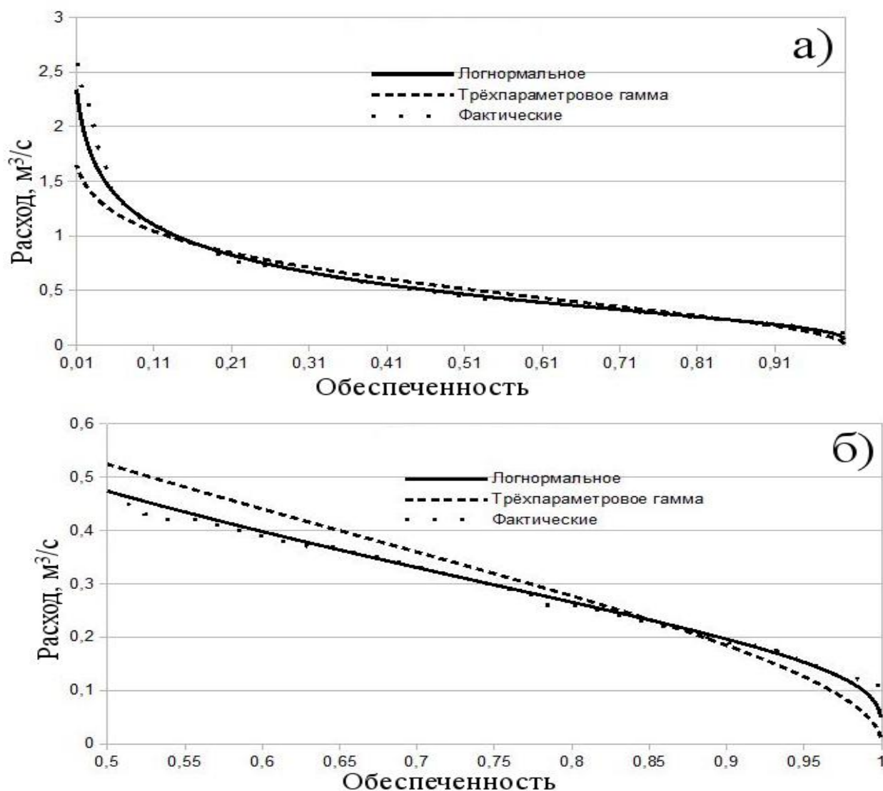
Рис. 2. а) кривая обеспеченности суточных расходов воды по посту Малый Черемшан-Абалдуювка; б) фрагмент правой части кривой
