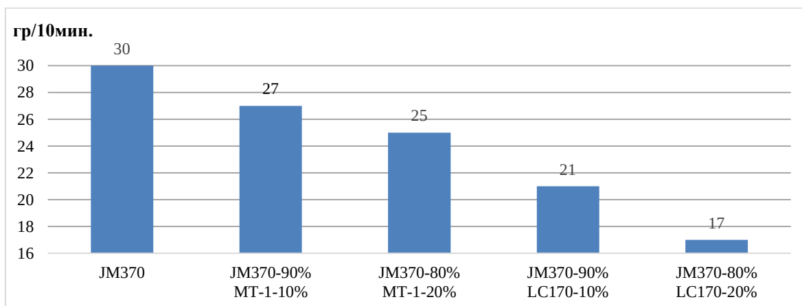
Рисунок 2. Зависимость ПТР компаунда от содержания талька и эластомера
