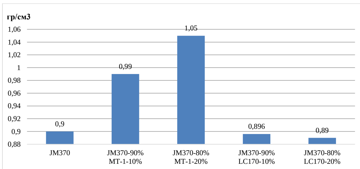
Рисунок 1. Зависимость плотности компаунда от содержания талька и эластомера
