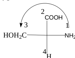
(S)-2-амино-3-гидроксипропановая к-та
