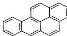
бензпирен
