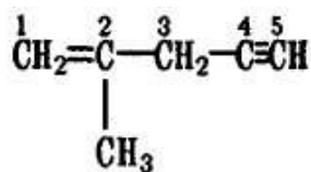
2-метилпентен-1-ин-4
