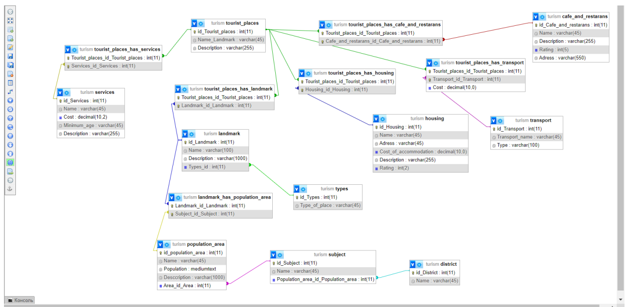
Рисунок 2.1 – Логическая схема
