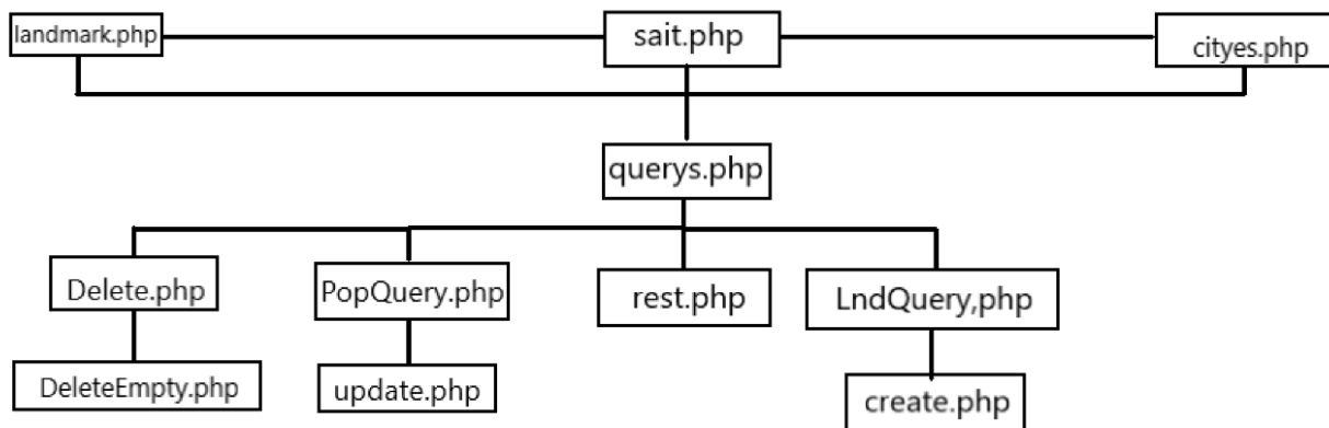
Рисунок 4 – структура приложения
