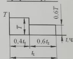
График нагрузки
