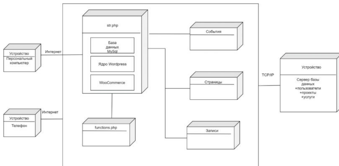
Рисунок 20 - UML-диаграмма развертывания
