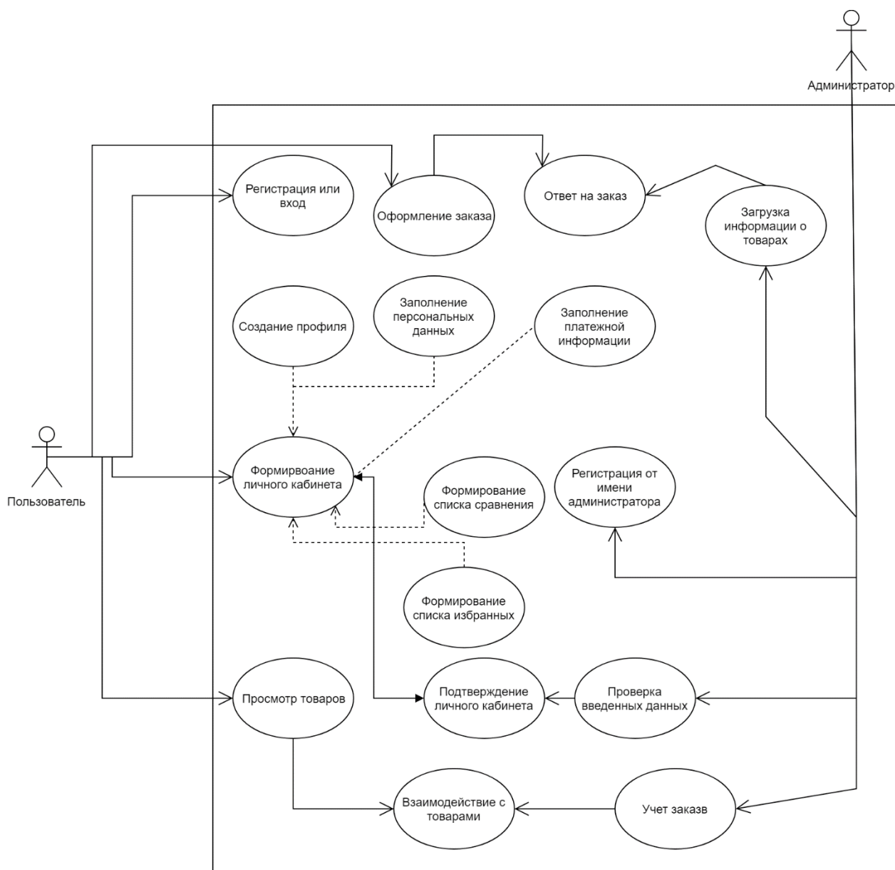
Рисунок 2 – UML -диаграмма вариантов использования
