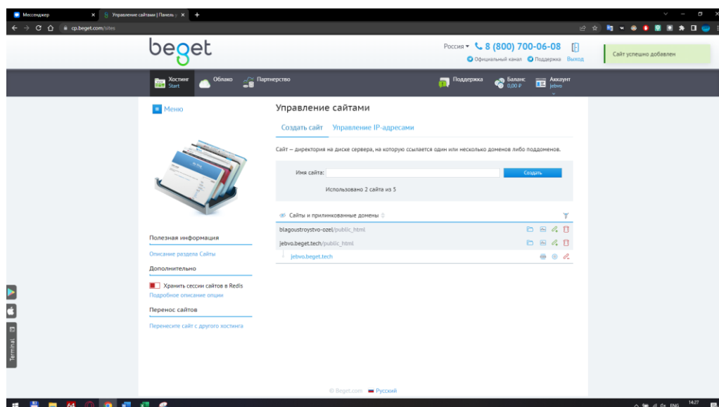
Рисунок 7 – Привязанный домен
