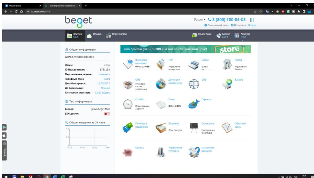
Рисунок 5 – Панель администрирования
