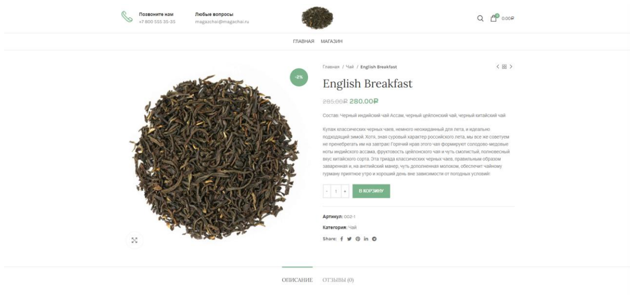
Рисунок 10 – Просмотр товаров
