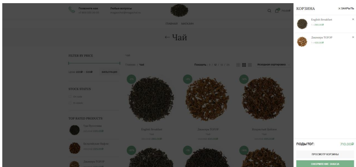
Рисунок 13 – Корзина
