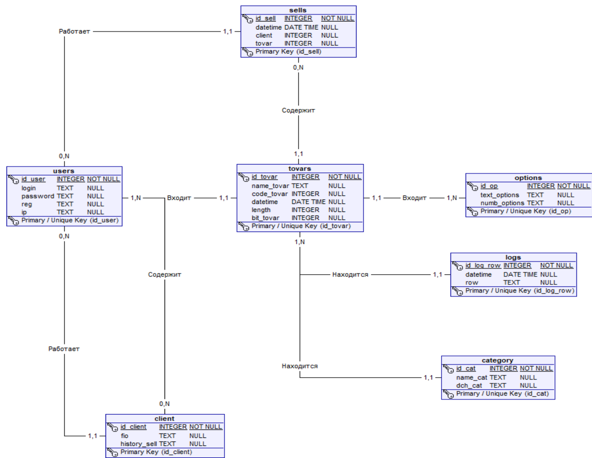
Рисунок 8 - Схема таблиц
