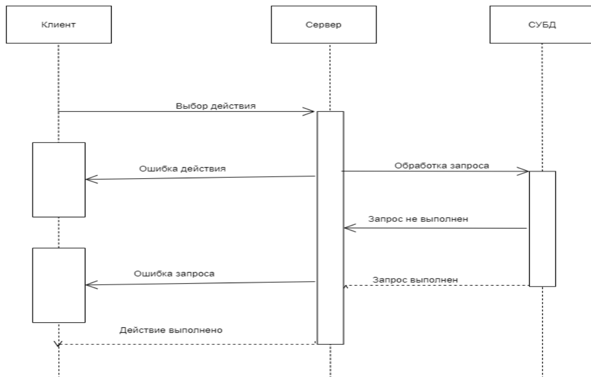
Рисунок 1 – UML-диаграмма последовательностей
