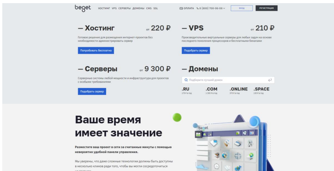
Рисунок 4 – Регистрация
