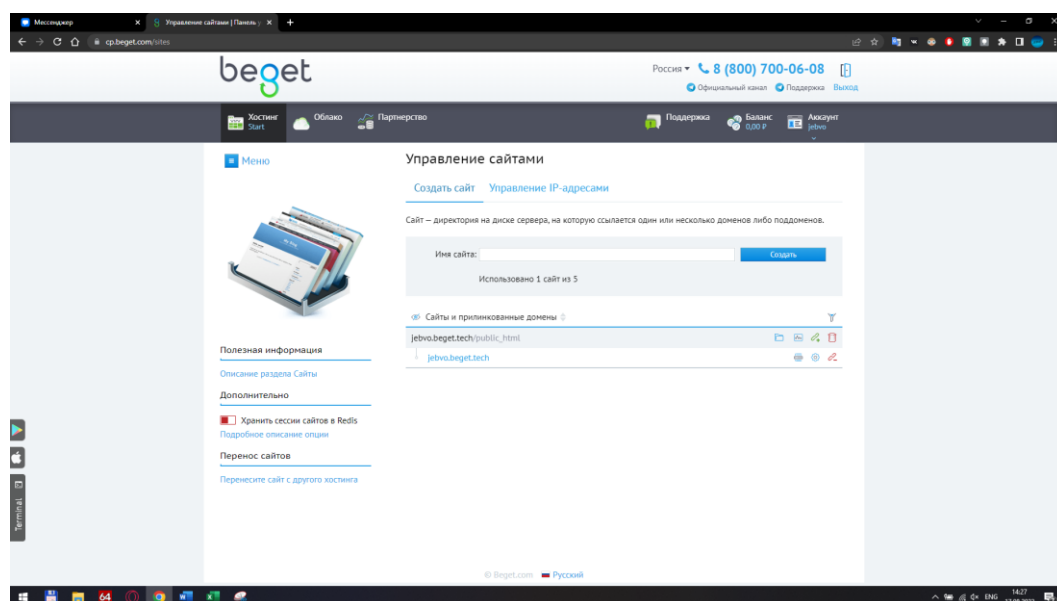
Рисунок 6 – Создание сайта
