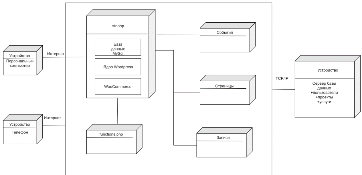
Рисунок 20 - UML-диаграмма развертывания
