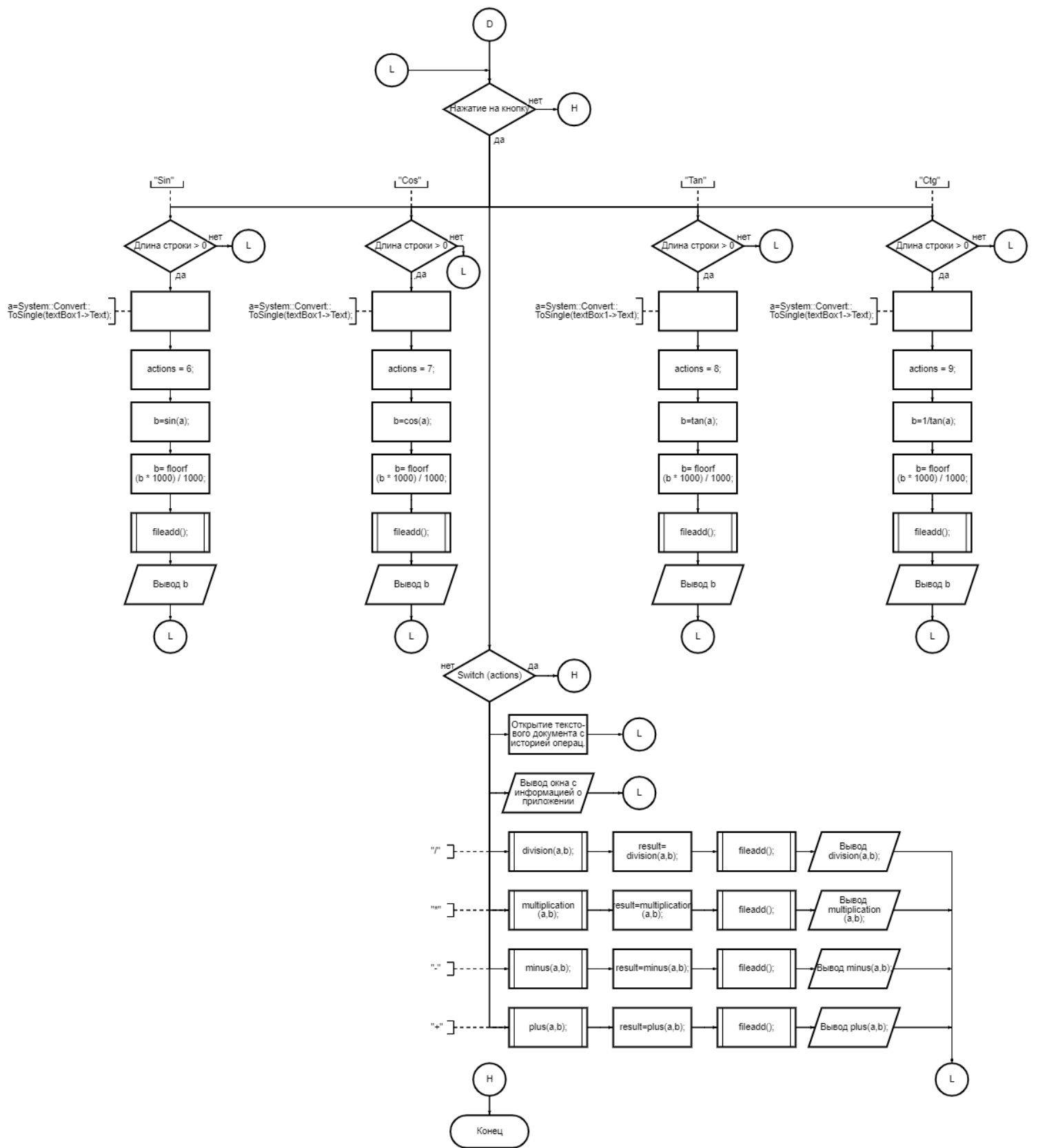
Рисунок – класс Form1
