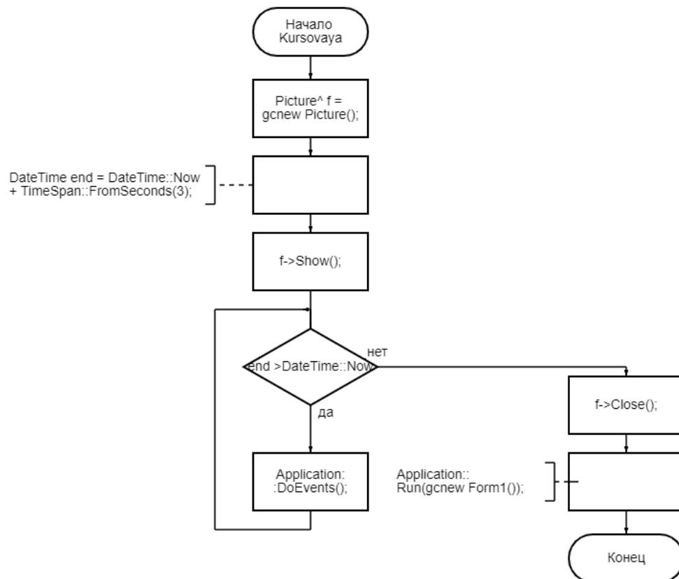
Рисунок – функция Kursovaya
