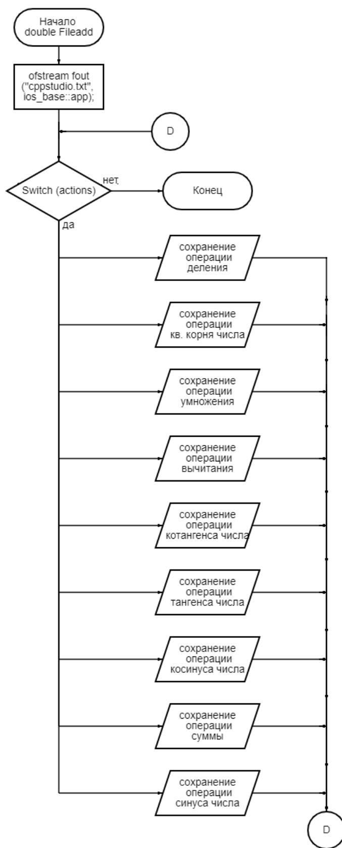
Рисунок – функция FileAdd
