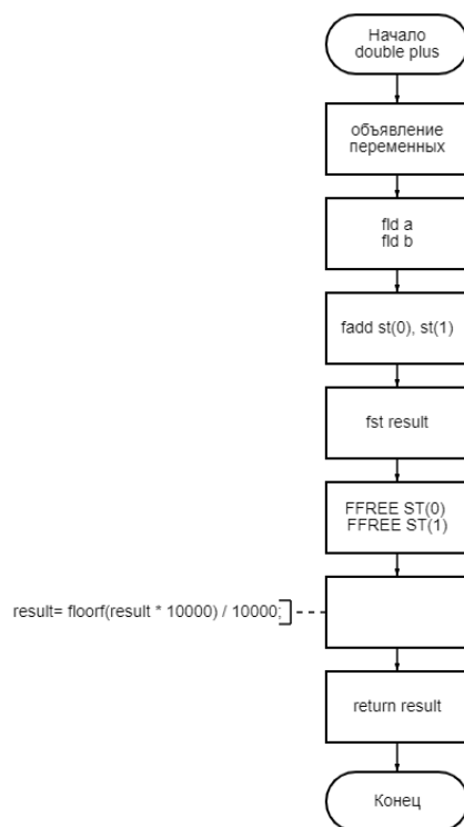
Рисунок – функция plus
