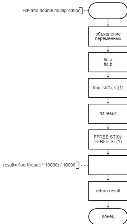
Рисунок – функция multiplication
