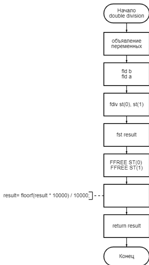
Рисунок – функция division
