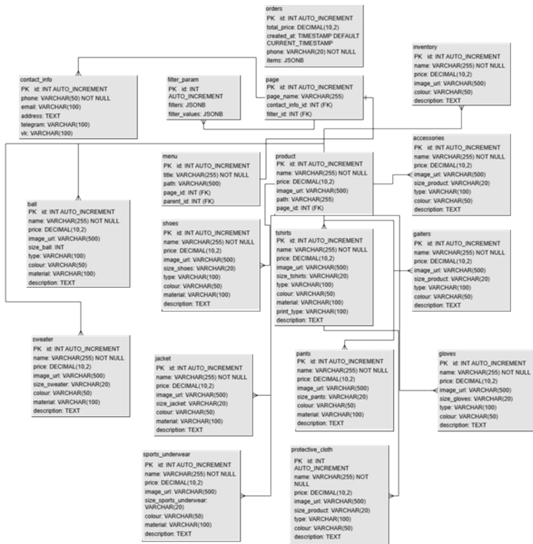
UML – диаграмма БД
