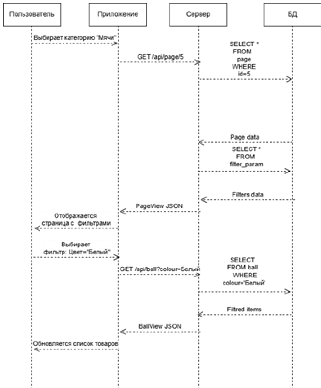
UML – диаграмма взаимодействия
