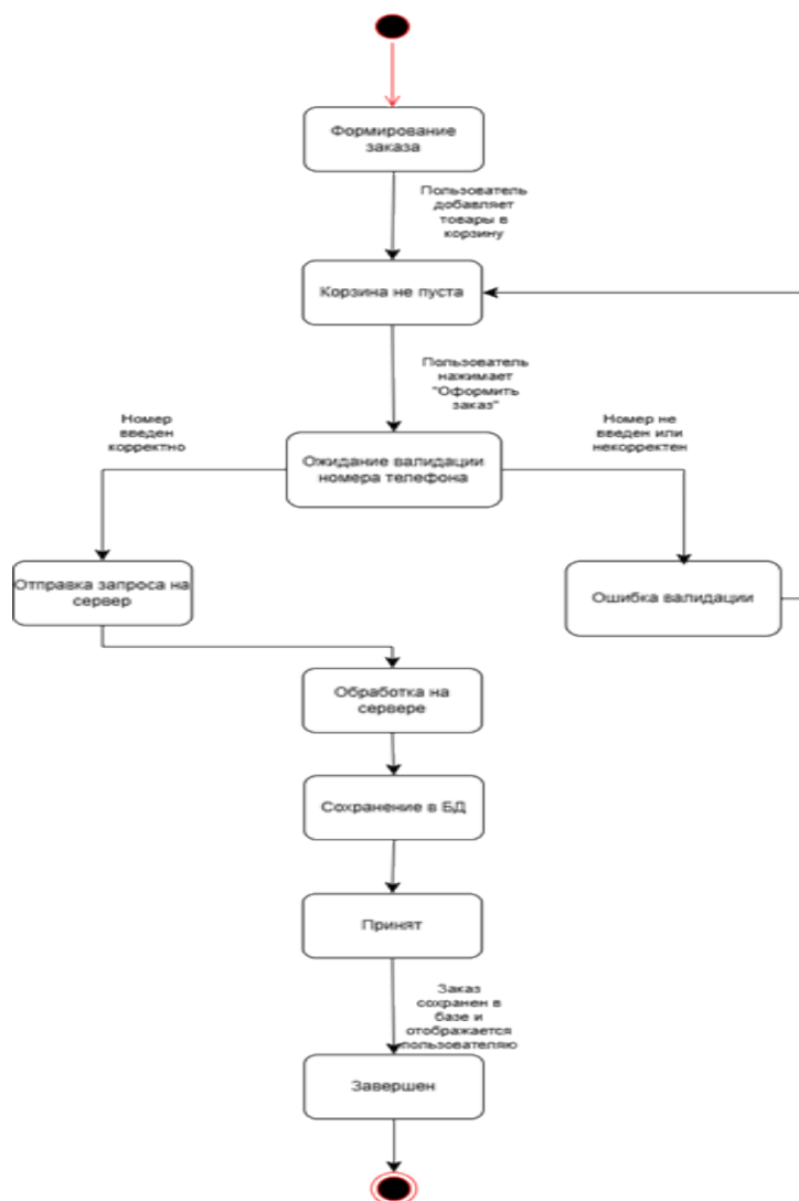
UML – диаграмма состояний
