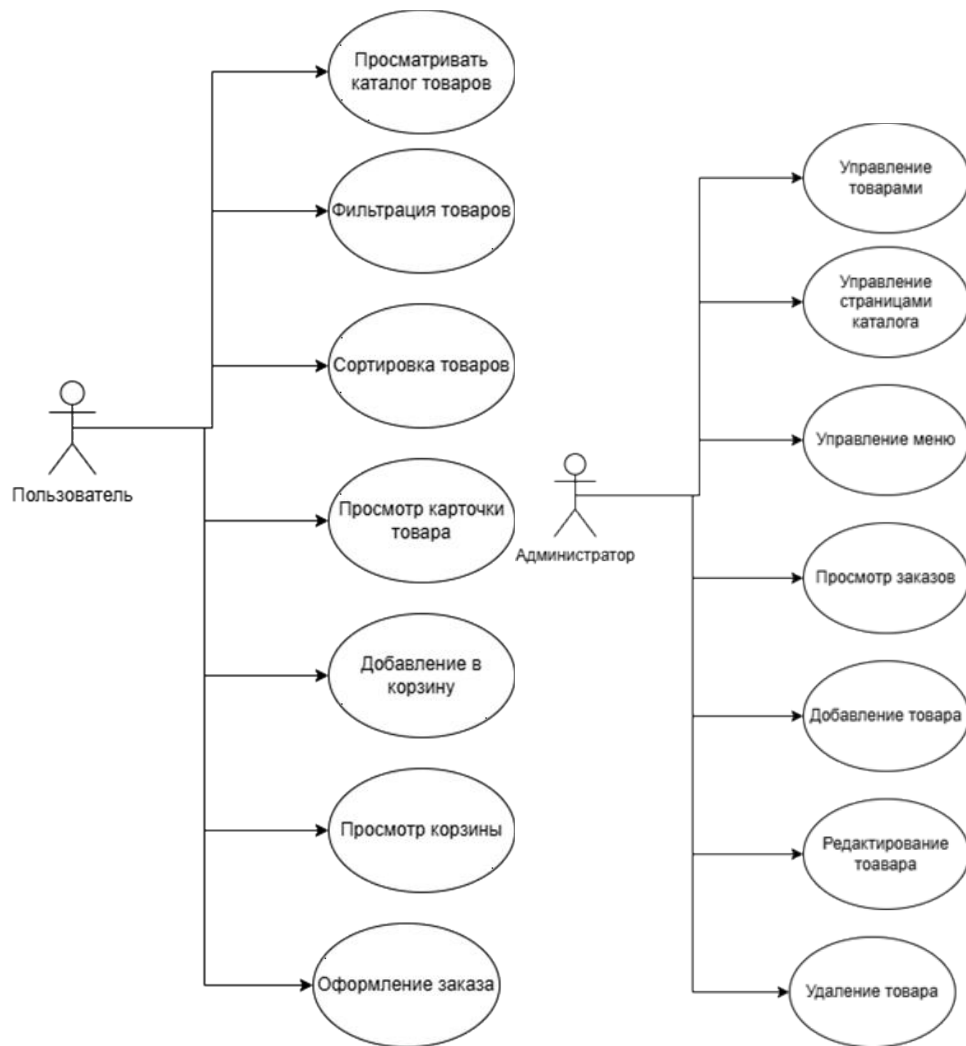
UML – диаграмма вариантов использования
