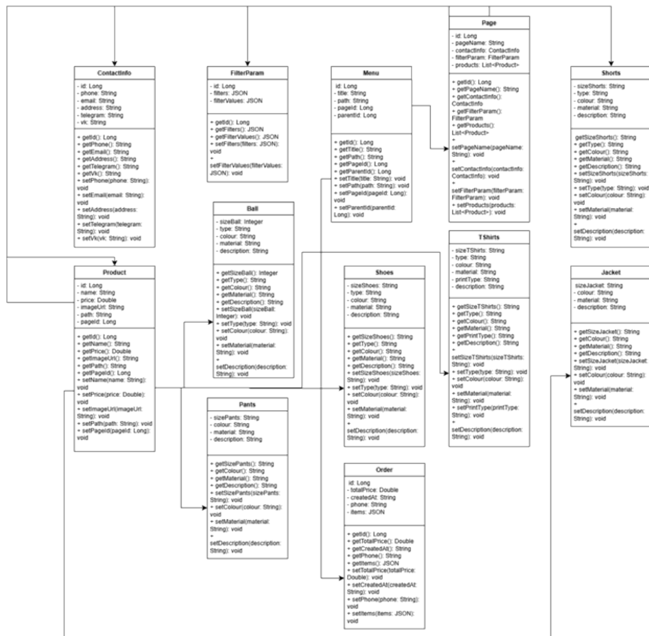
UML – диаграмма классов
