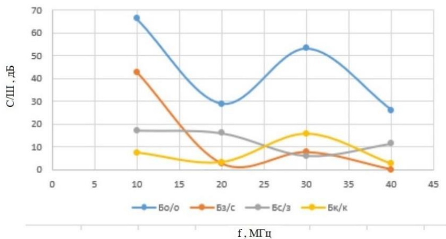
Рисунок 69 – Зависимость уровня сигнал/шум от частоты для жил кабеля типа UTP
