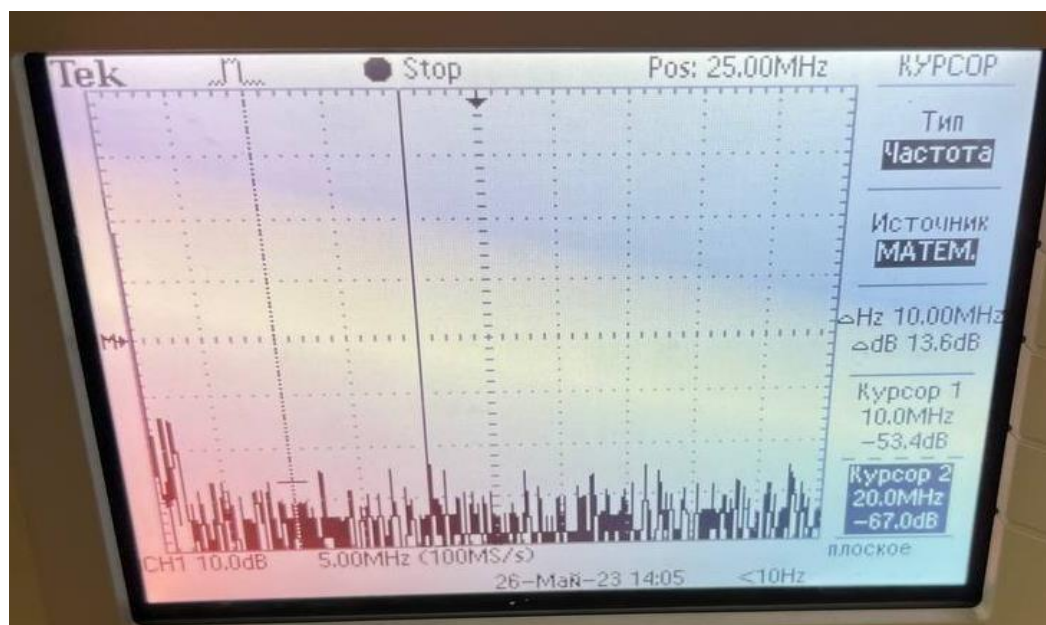
Рисунок 43 – Показания осциллографа в 16 эксперименте
