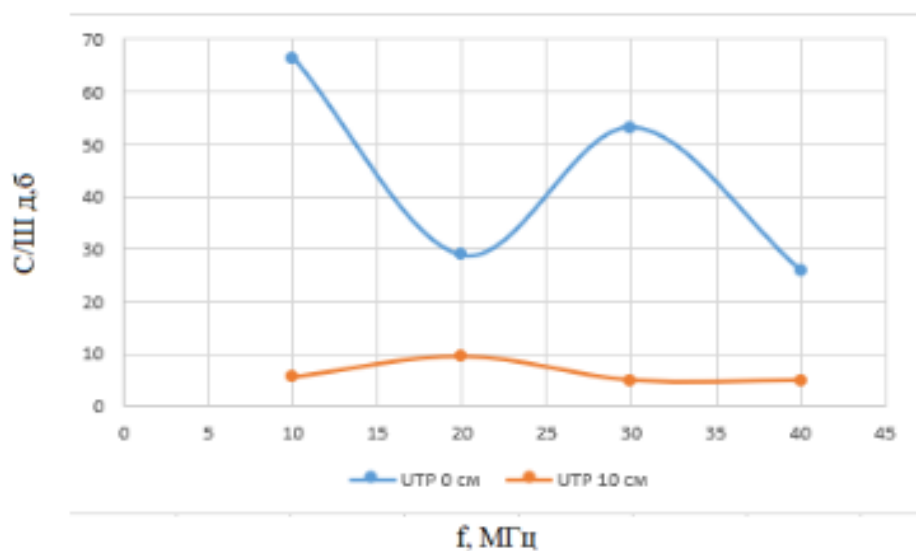
Зависимость уровня сигнал/шум от частоты для кабеля типа UTP
