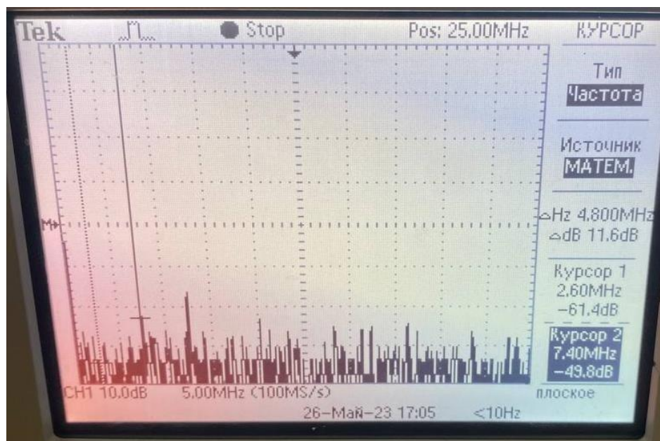
Рисунок 63 – Показание осциллографа в 35 эксперименте
