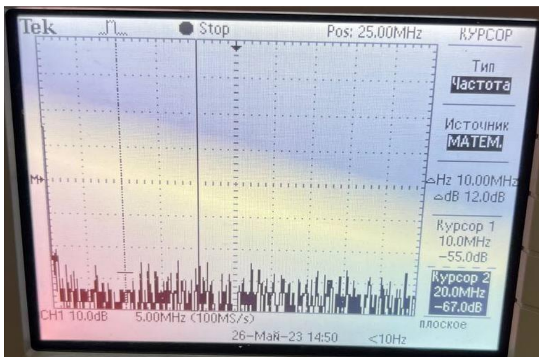
Рисунок 48 – Показание осциллографа в 21 эксперименте
