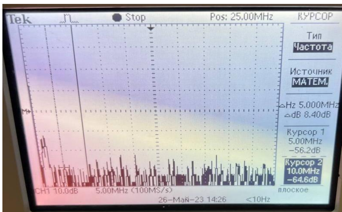
Рисунок 46 – Показание осциллографа в 19 эксперименте
