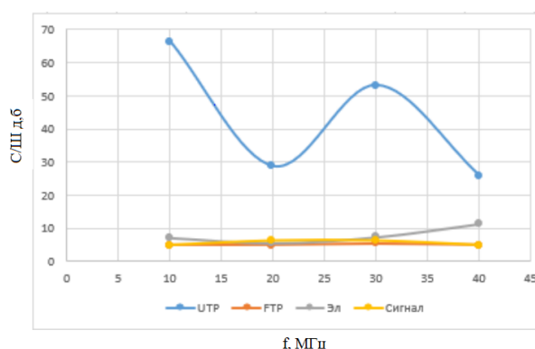
Зависимость уровня сигнал/шум от частоты для кабелей всех типов кабельном канале
