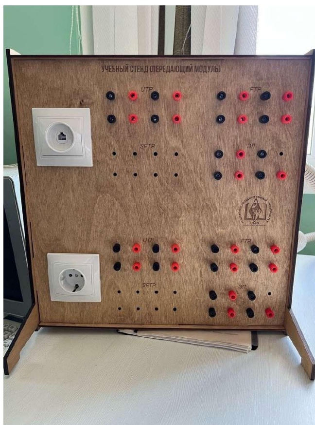
Рисунок 9 – Передающий модуль стенда.
