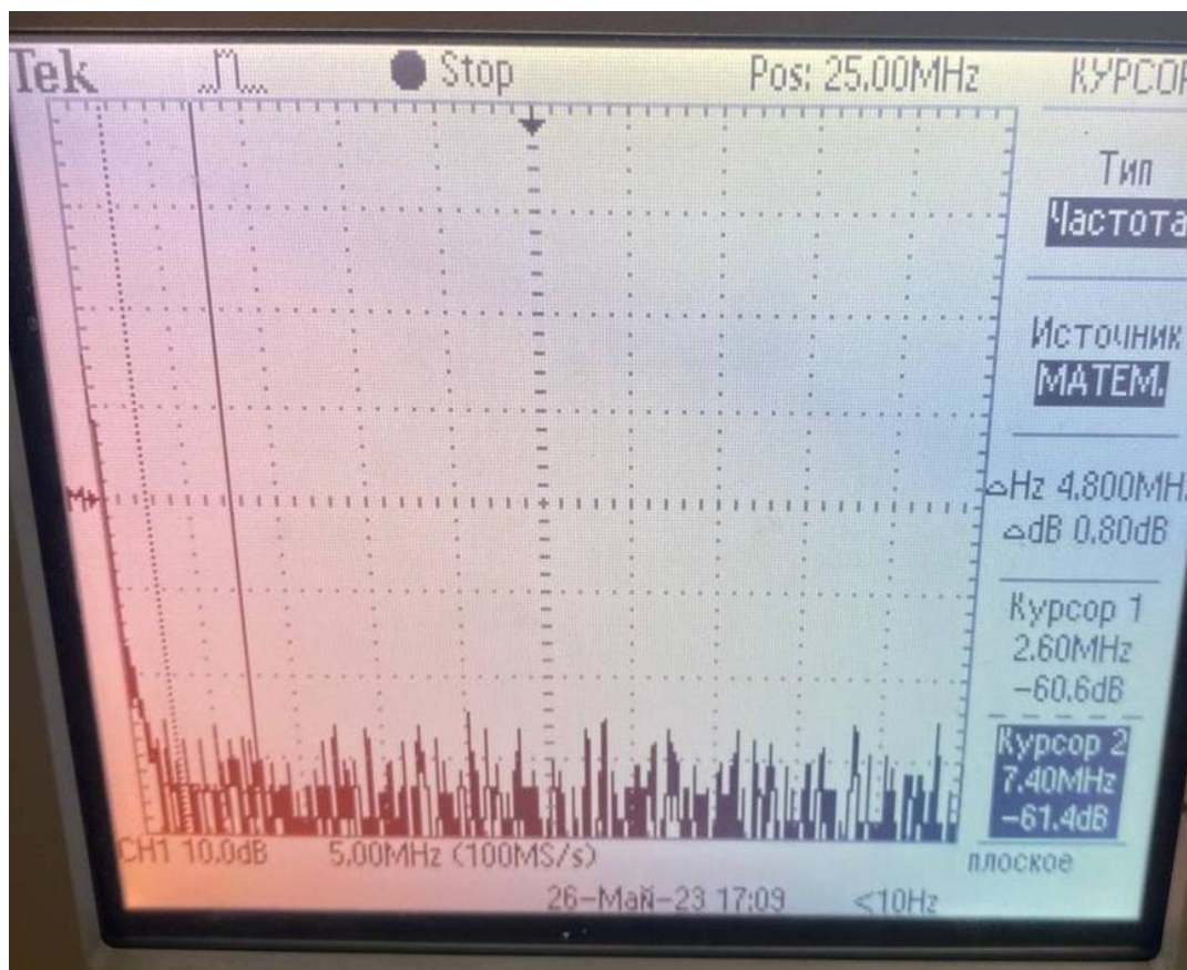
Рисунок 68 – Показание осциллографа в 40 эксперименте
