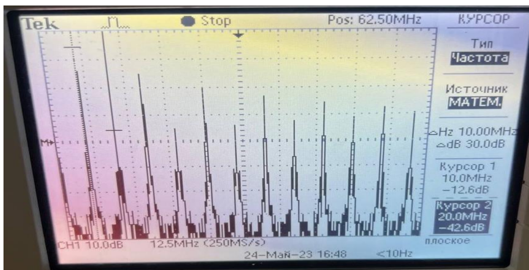
Рисунок 27 – Показание осциллографа в 1 эксперименте
