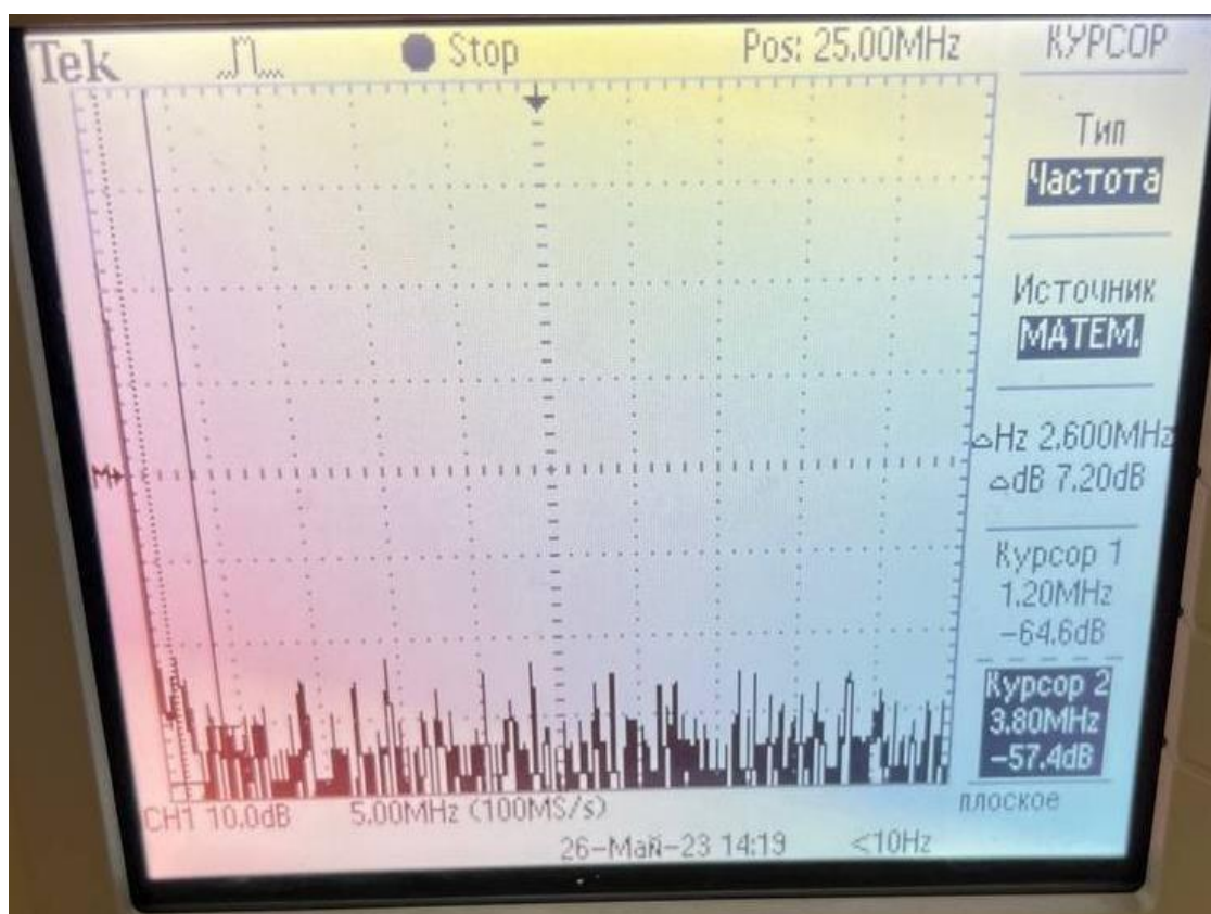
Рисунок 45 – Показание осциллографа в 18 эксперименте
