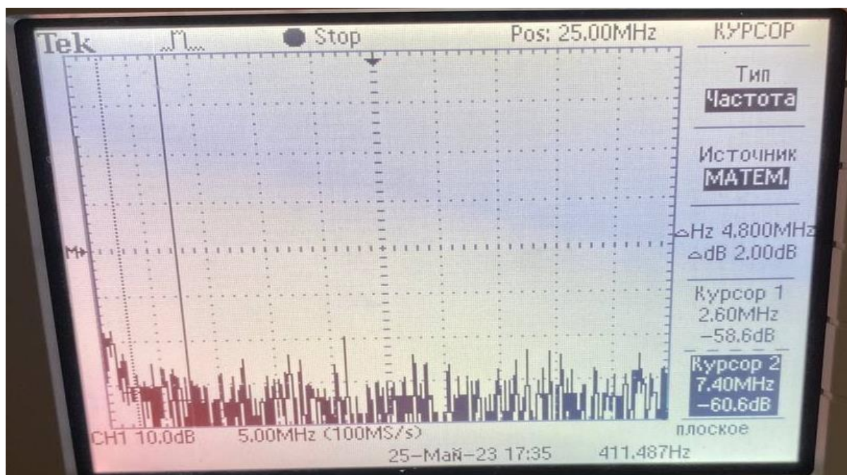
Рисунок 42 – Показание осциллографа в 15 эксперименте Результаты эксперимента 15 были сведены в таблицу 16.
