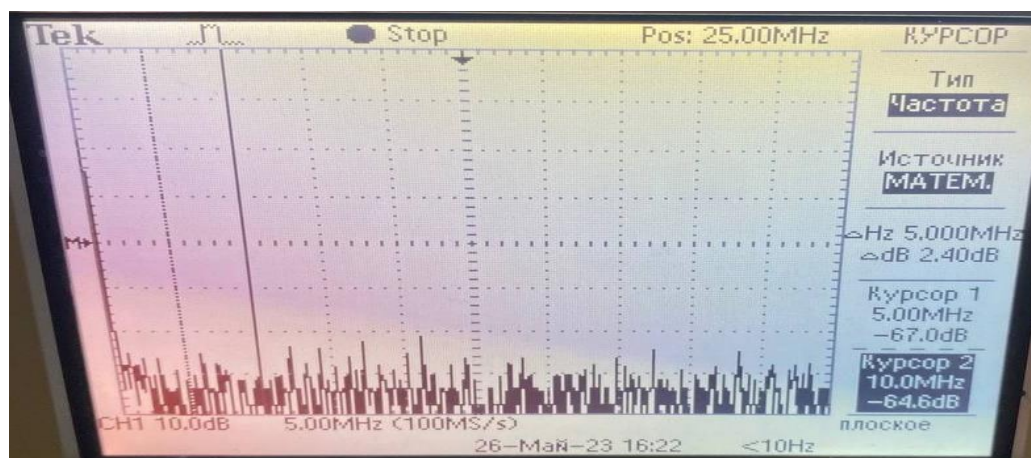
Рисунок 50 – Показание осциллографа в 23 эксперименте
