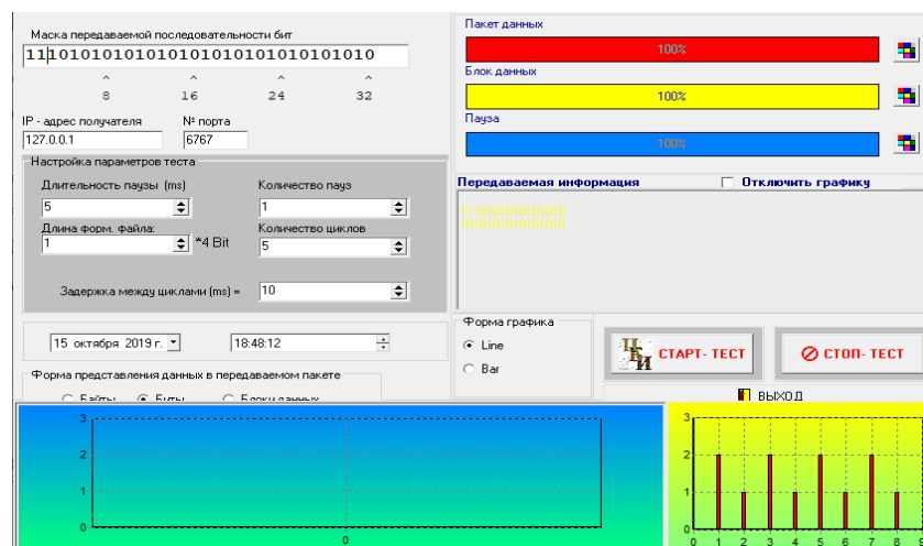
Рисунок 7 – Окно программы UDPtest
