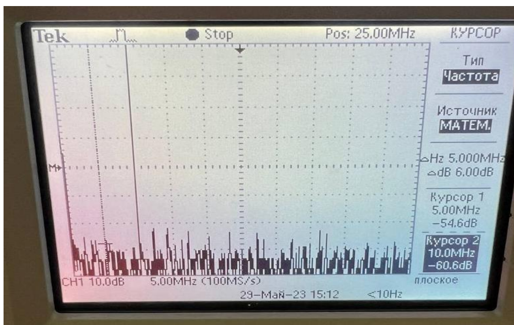
Рисунок 55 – Показание осциллографа в 28 эксперименте
