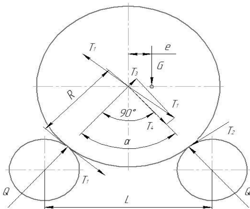
Рисунок 21 - Расчетная схема стэнда с роликовым подшипником
