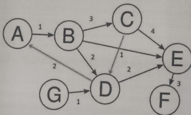
Рисунок 1 – Пример орграфа
