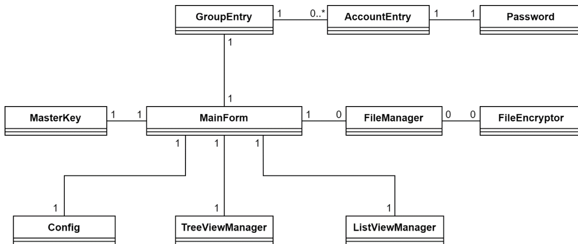
Рисунок 1.12 – UML-диаграмма объектов
