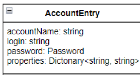
Рисунок 1.9 – Поля и методы класса AccountEntry
