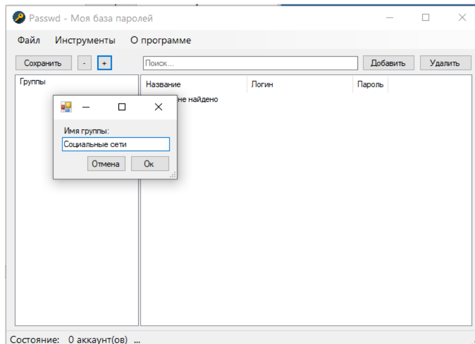
Рисунок 1.16 – Создание группы
