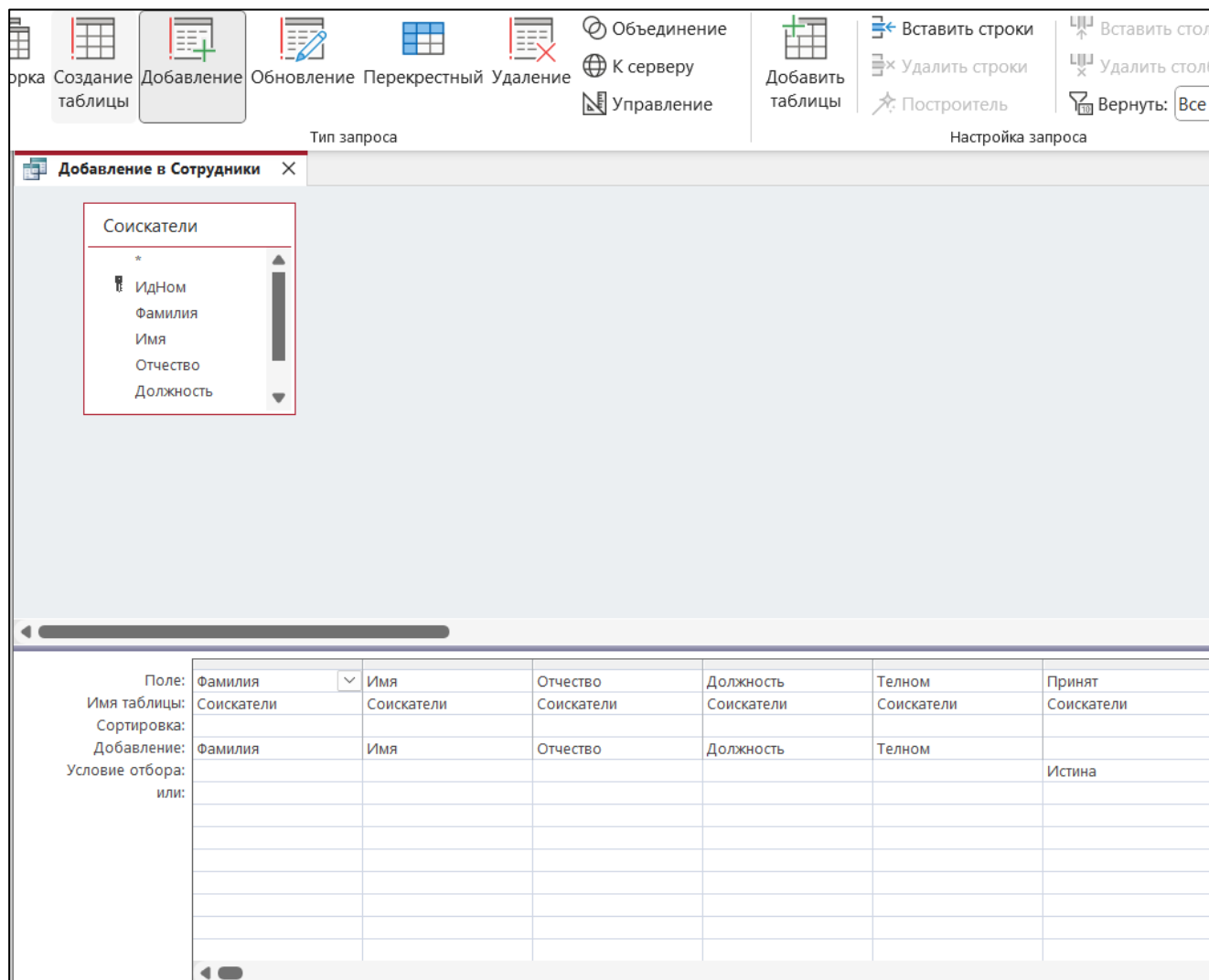
Рисунок Е.1 – Запрос на добавление информации о принятых соискателя в таблицу Сотрудники
