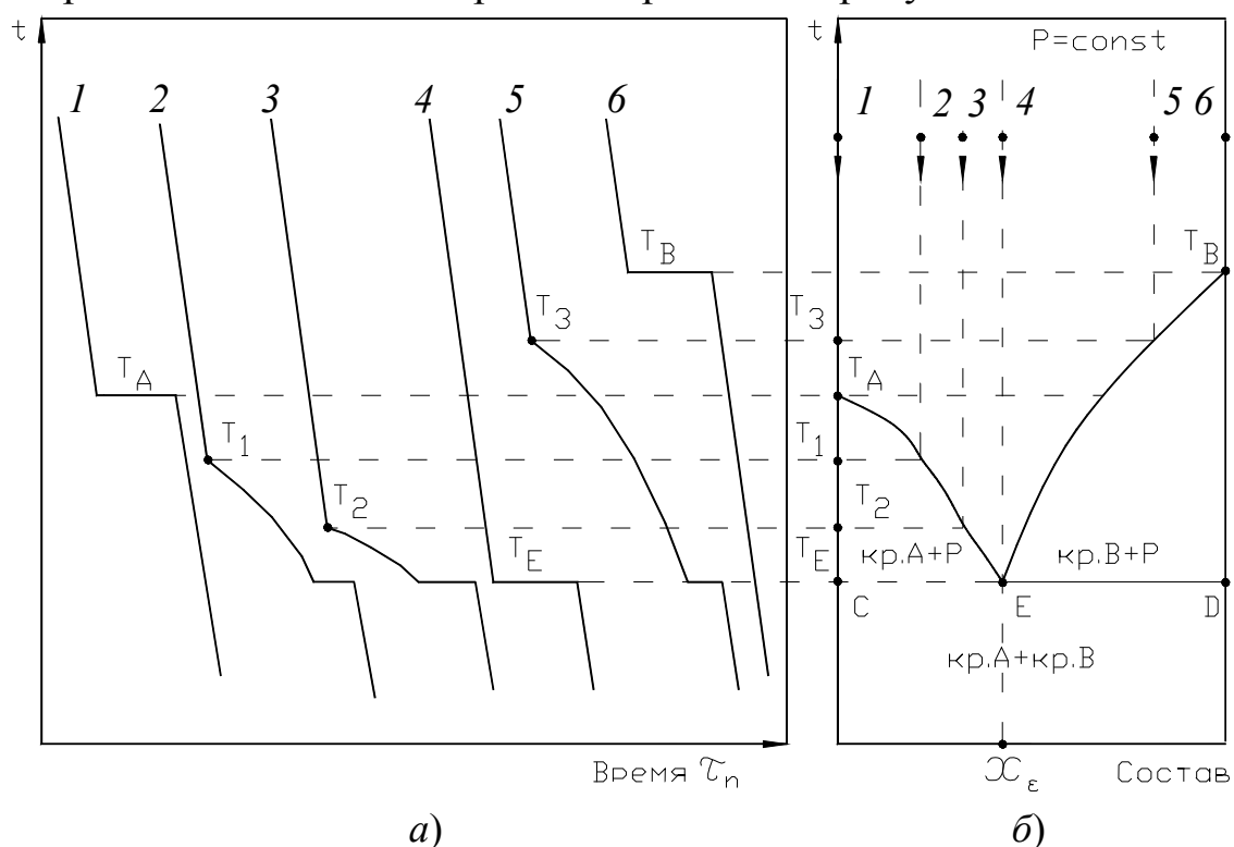
Кривые охлаждения (а) и диаграмма плавкости (б) неизоморфной смеси без образования химических соединений
