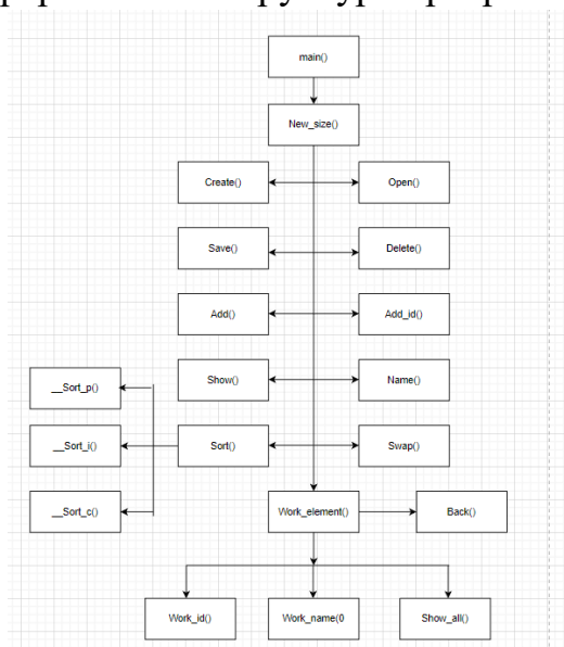
Рисунок 4 — структура данных
