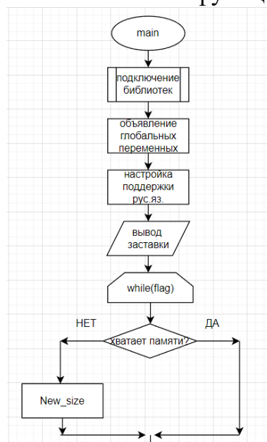
рисунок 4 - Схема данных
