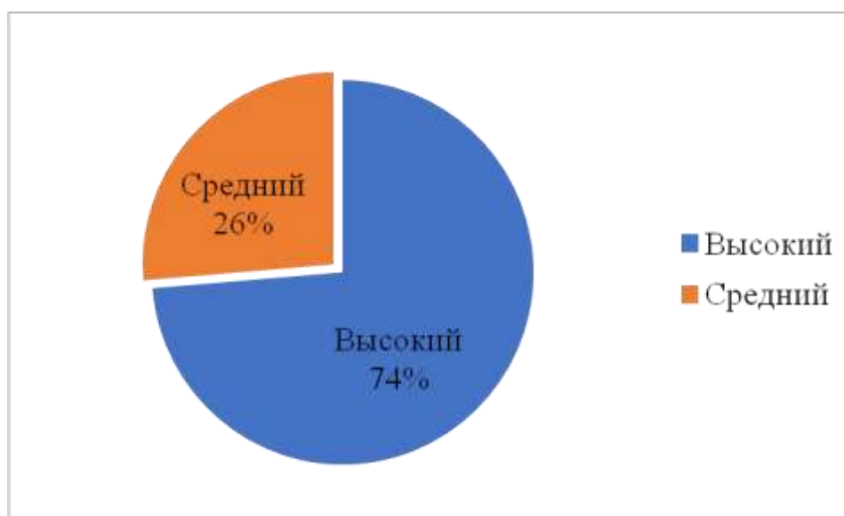
Рис. 5. Анализ рассказа
