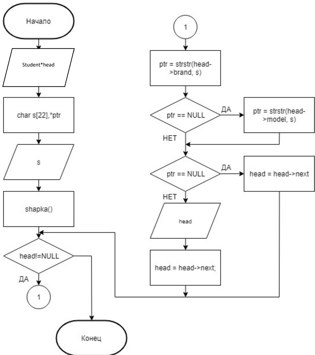
Рисунок 14 - функция поиска
