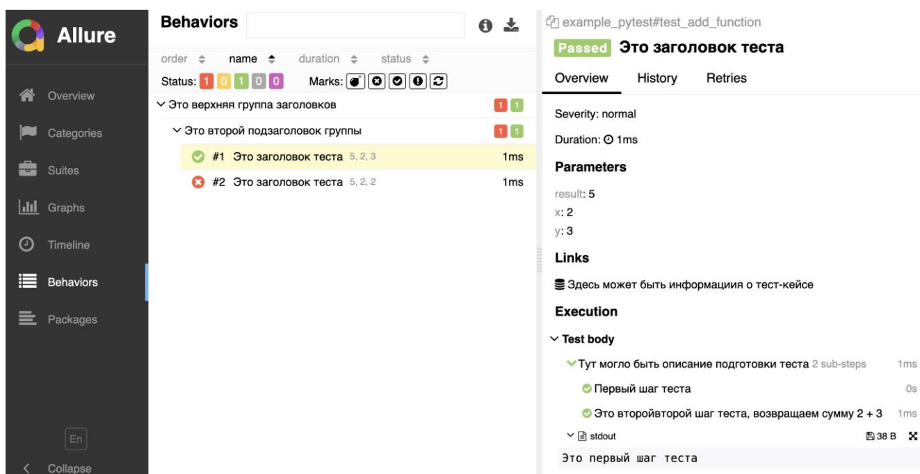
Рисунок 9 – Пример отчета о прохождении теста с форматированием Allure
