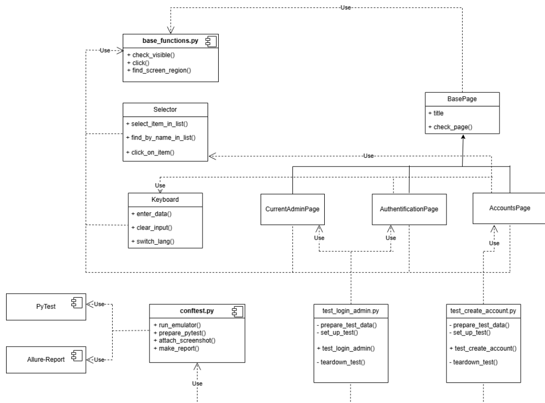
Рисунок 13 – Диаграмма классов проекта авто–тестов
