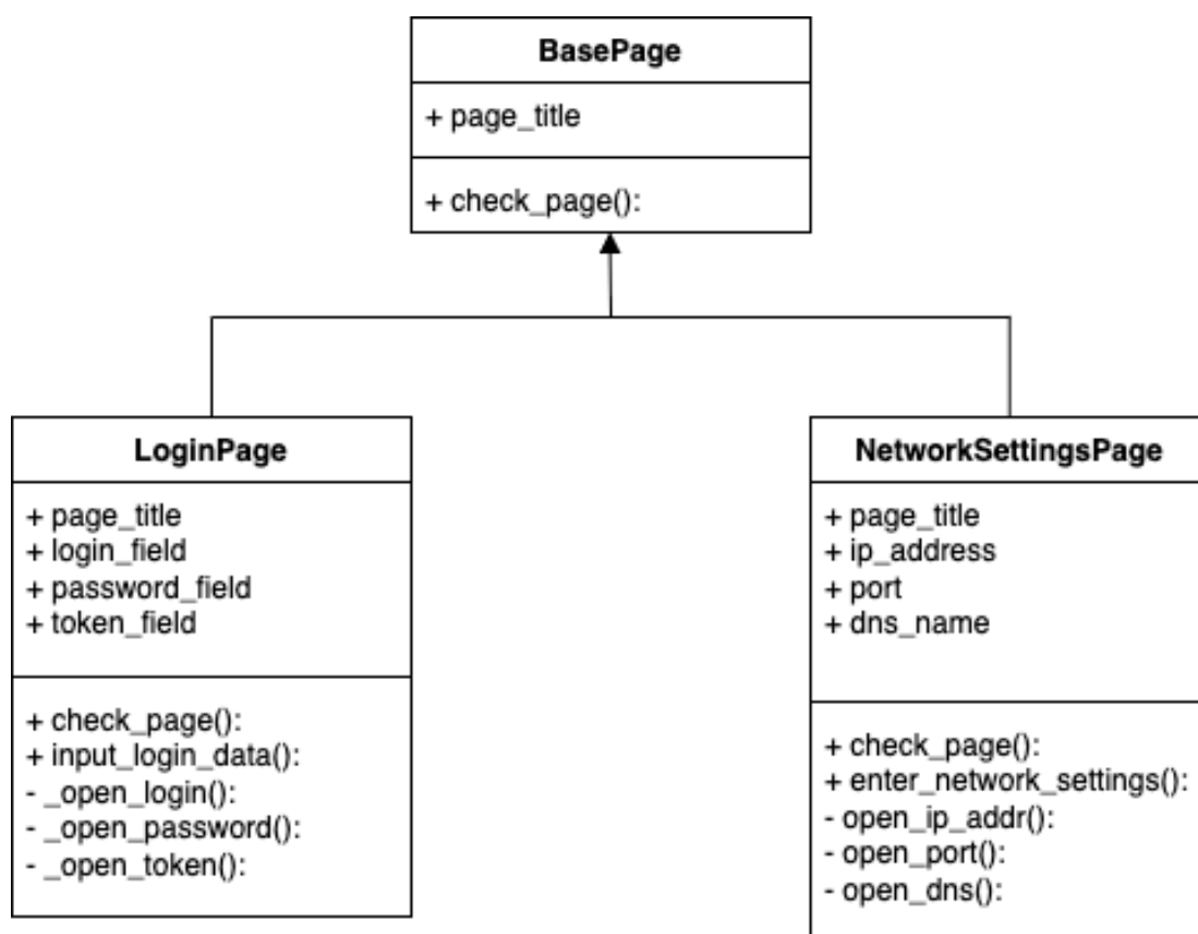
Рисунок 19 – UML-диаграмма классов страниц согласно паттерну PageObject
