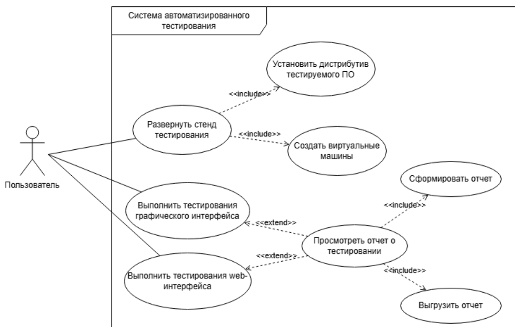
Рисунок 5 – Диаграмма вариантов использования
