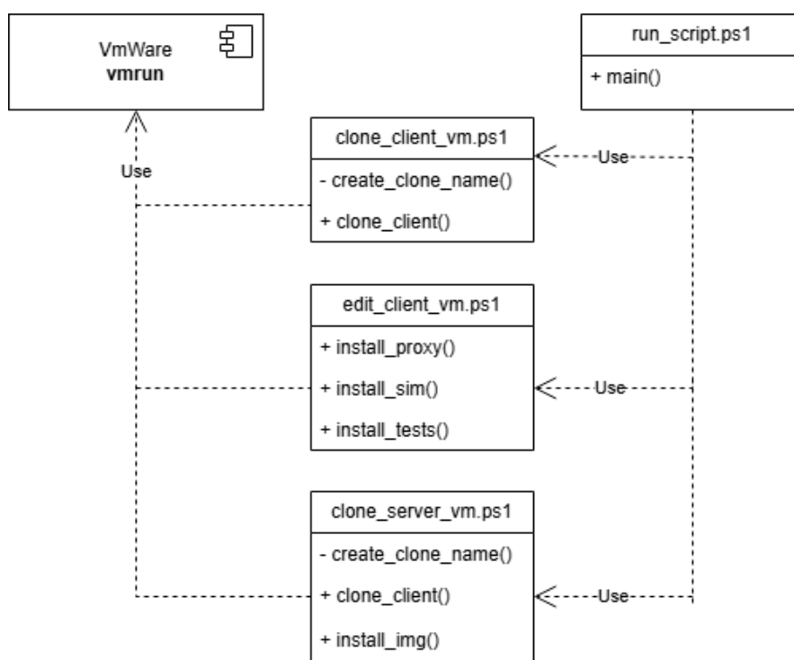
Рисунок 14 – Диаграмма классов автоматического развертывания стенда
