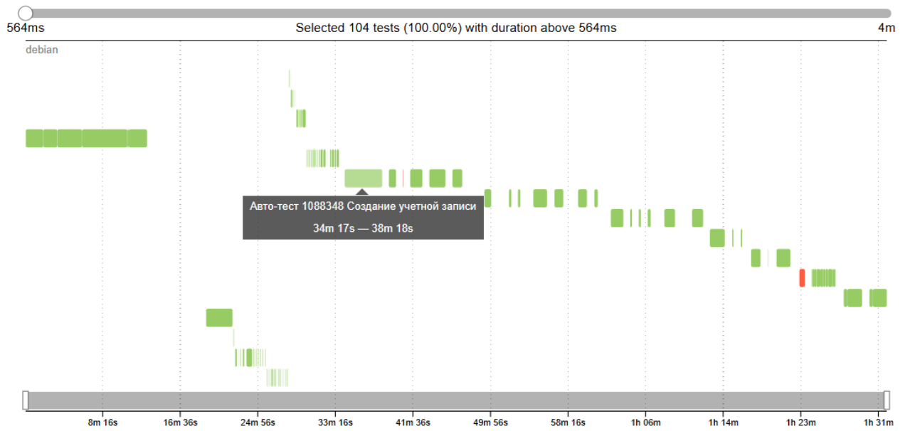
Рисунок Г.3 – Временной график прохождения авто-тестов
