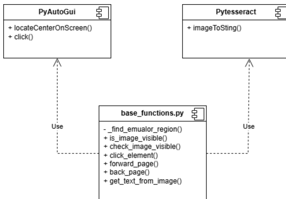
Рисунок 12 – Диаграмма классов базового функционала
