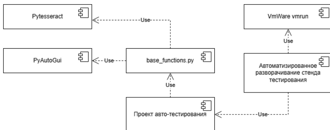
Рисунок 11 – Диаграмма компонентов системы тестирования
