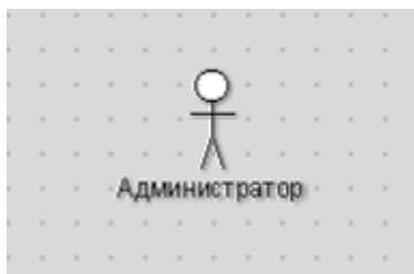
Рис. 2.1. Актер
