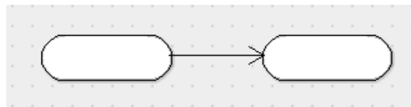
Рис. 3.4. Простой переход
