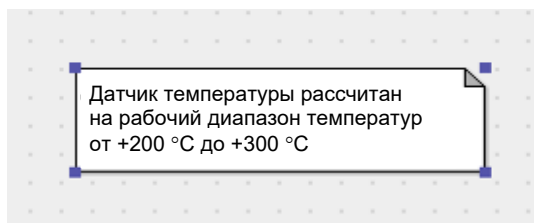
Рис. 2.4. Примечание
