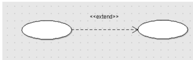
Рис. 2.6. Отношение расширения
