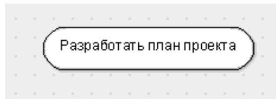
Рис. 3.3. Состояние действия
