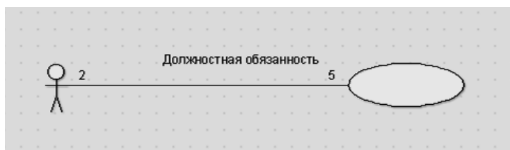
Рис. 2.5. Отношение ассоциации
