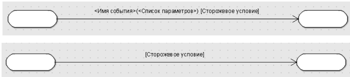
Рис. 3.6. Сторожевое условие
