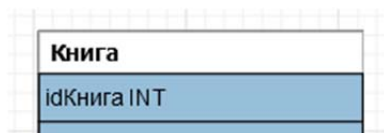
Рис. 5.3. Ключ
