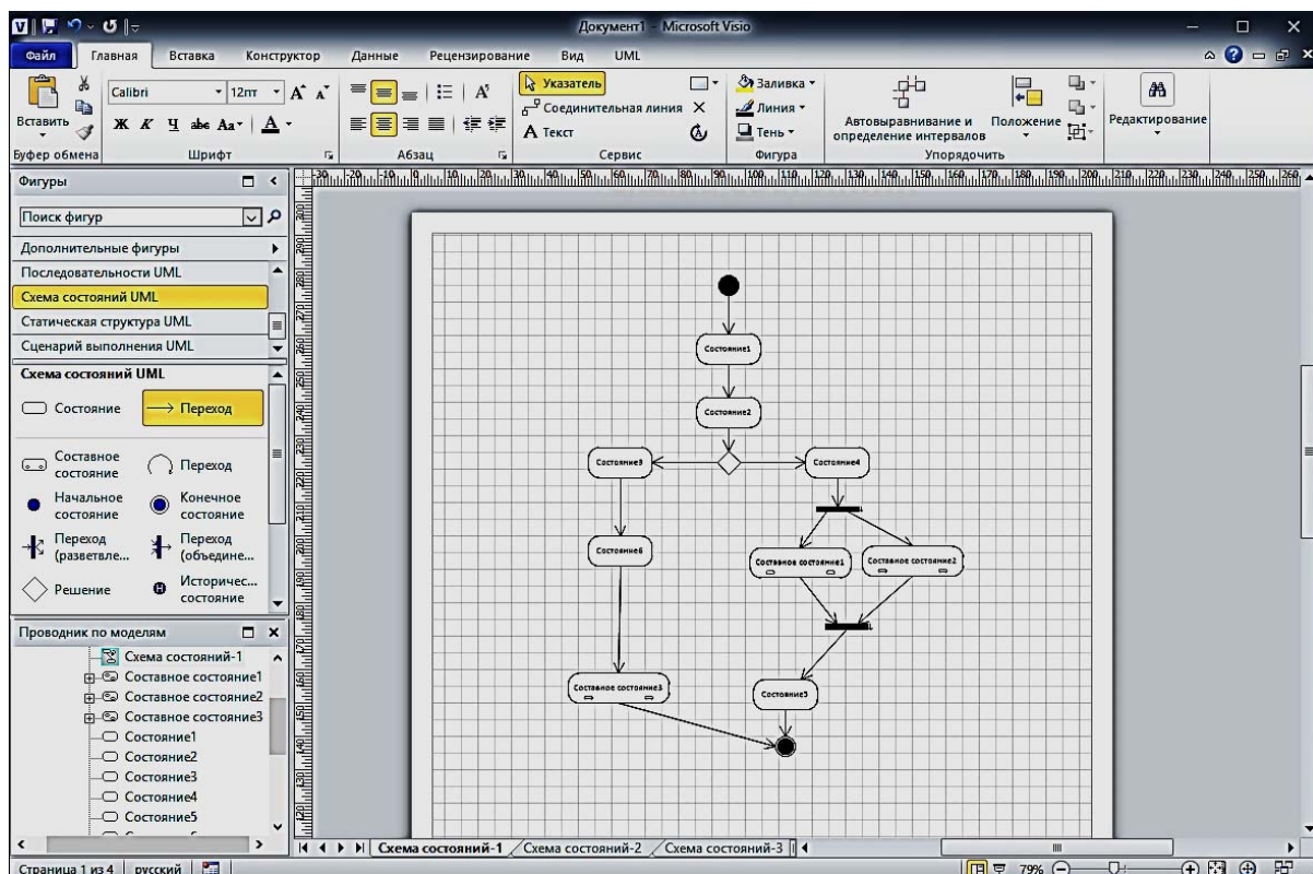
Рис. 3.12. Интерфейс Visio
