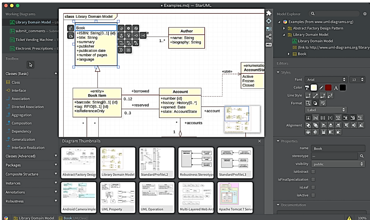
Рис. 2.9. Интерфейс StarUML
