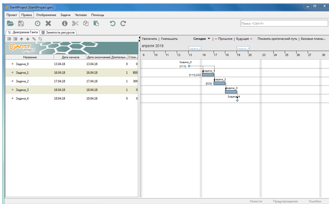
Рис. 6.9. Интерфейс GanttProject
