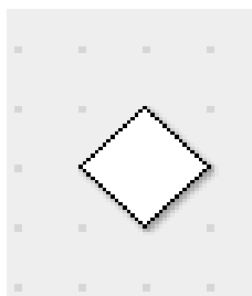
Рис. 3.8. Ветвление
