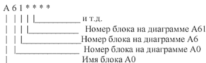
Рис. 4.8. Ссылочный код
