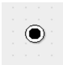
Рис. 3.2. Конечное состояние
