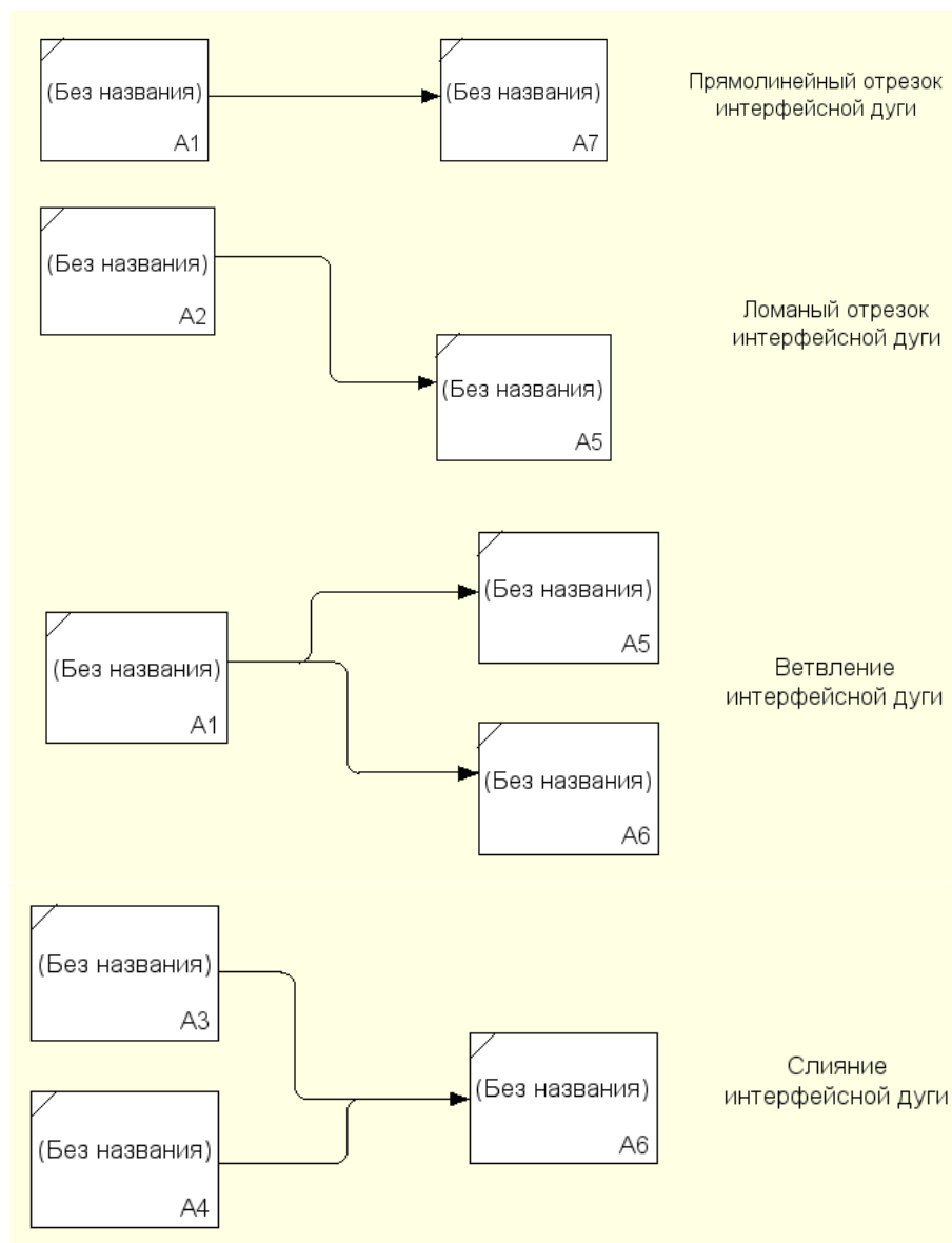
Рис. 4.2. Интерфейсная дуга
