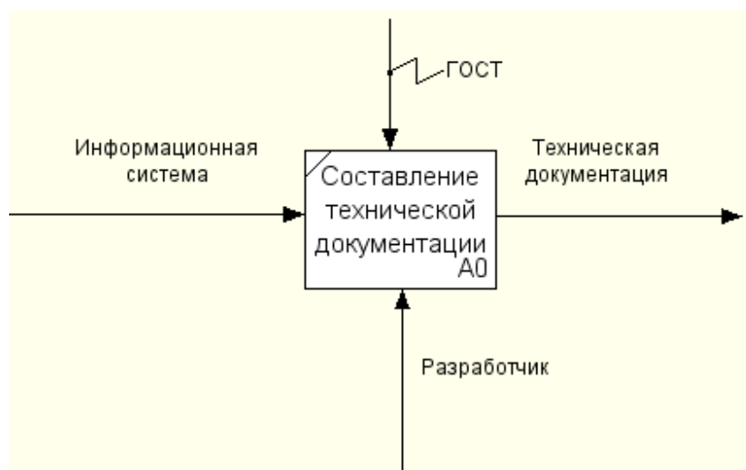
Рис. 4.6. Модель IDEF0
