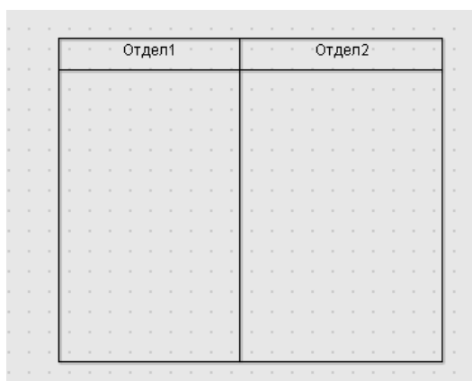
Рис. 3.10. Дорожки
