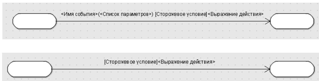
Рис. 3.7. Выражение действия
