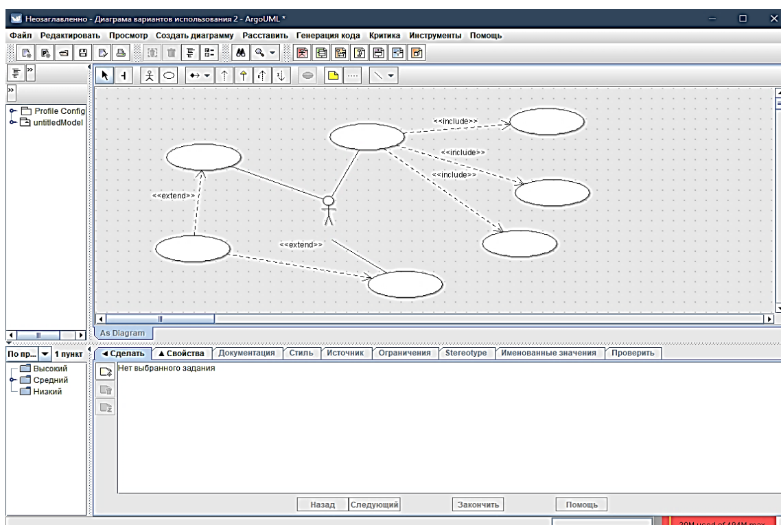
Рис. 2.10. Интерфейс ArgoUML
