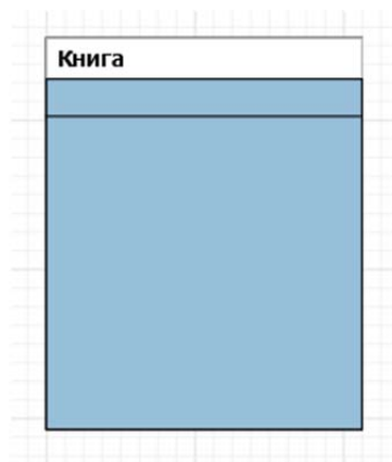
Рис. 5.1. Сущность
