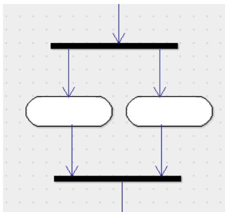
Рис. 3.9. Параллельные процессы
