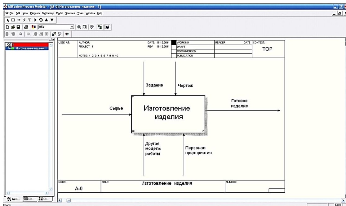
Рис. 4.16. Интерфейс AllFusion Process Modeler
