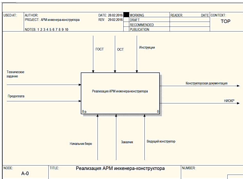
Рис. 4.7. Пример диаграммы А-0
