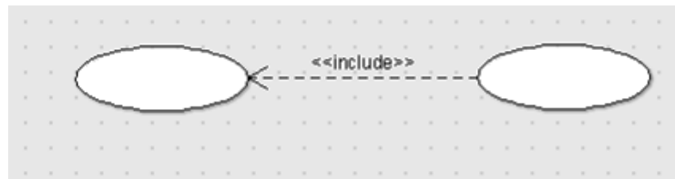
Рис. 2.7. Отношение включения
