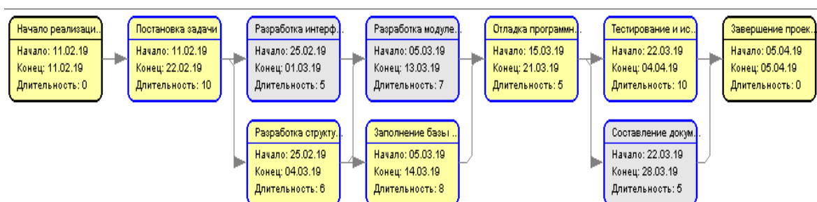
Рис. 6.4. PERT-диаграмма
