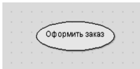
Рис. 2.2. Вариант использования
