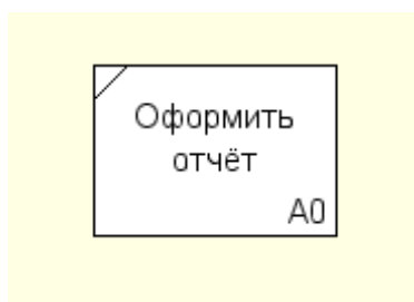
Рис. 4.1. Блок
