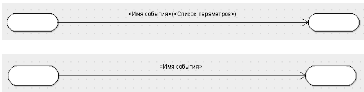
Рис. 3.5. Обозначение события
