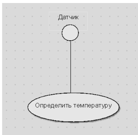
Рис. 2.3. Интерфейс
