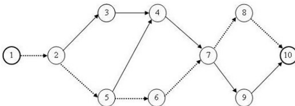
Рис. 6.3. Критический путь
