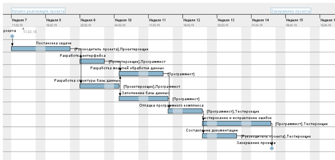
Рис. 6.6. Диаграмма Ганта
