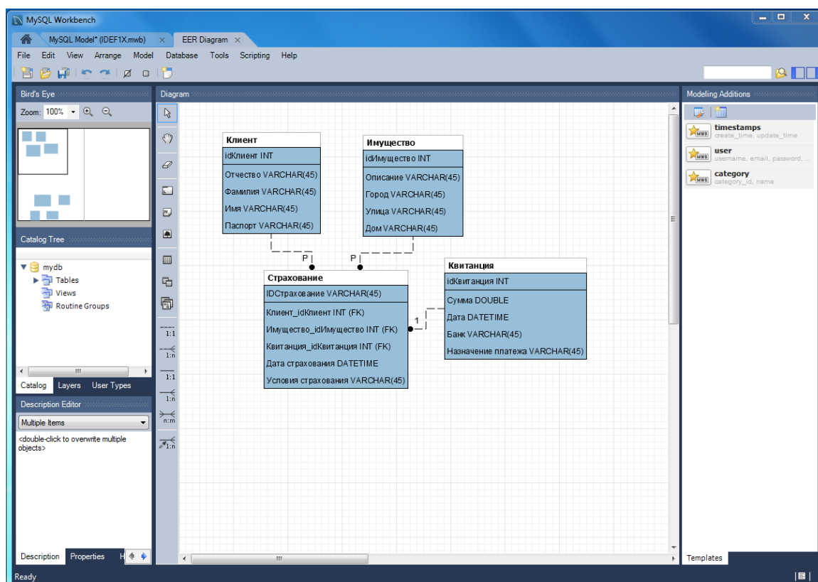
Рис. 5.10. Интерфейс MySQL Workbench
