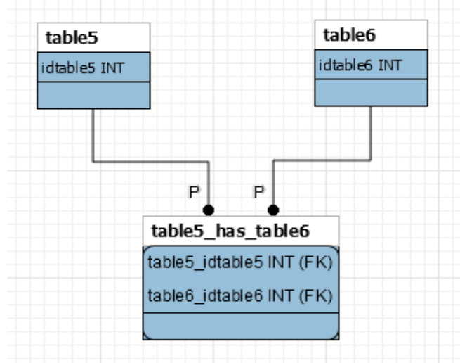
Рис. 5.7. Пример преобразования связи типа много-ко-многим
