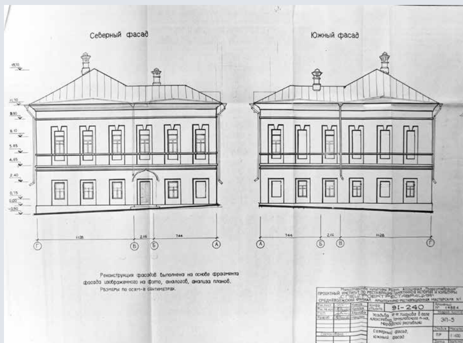
Графическая реконструкция северного и южного фасадов усадебного дома Ф. Ф. Ушакова. ЦГА РМ. Ф. Р-1122. Оп. 5. Д. 45. Л. 17
