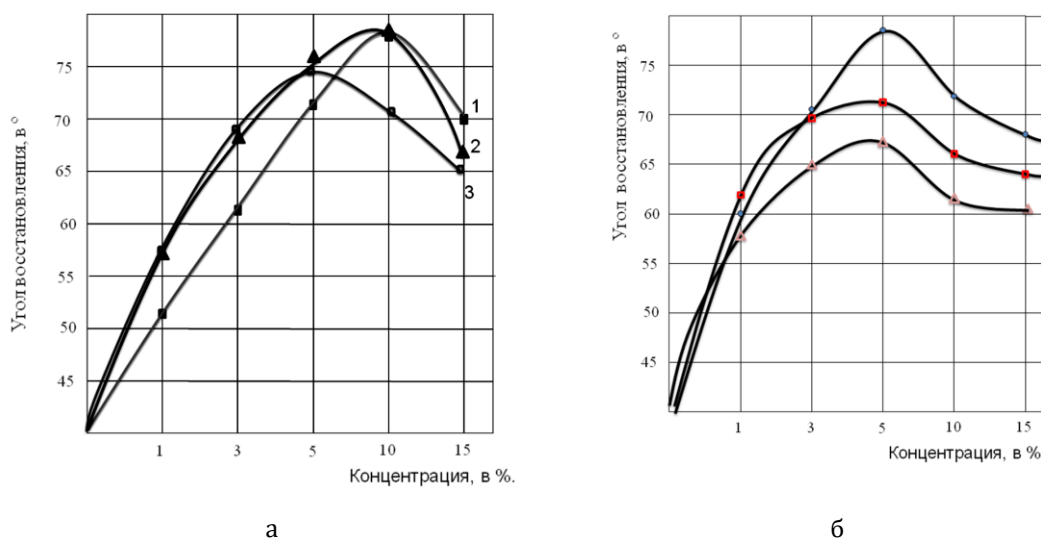
Рис. 1. Показатели углов восстановления по основе – (а) и утку – (б) в зависимости от условия сушки опытных образцов: 1 - естественная, 2 - контактная и 3 - конвективная
