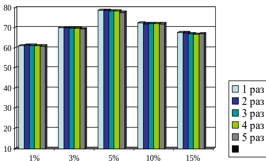
Рис. 3. Показатели углов восстановления после стирки по утку
