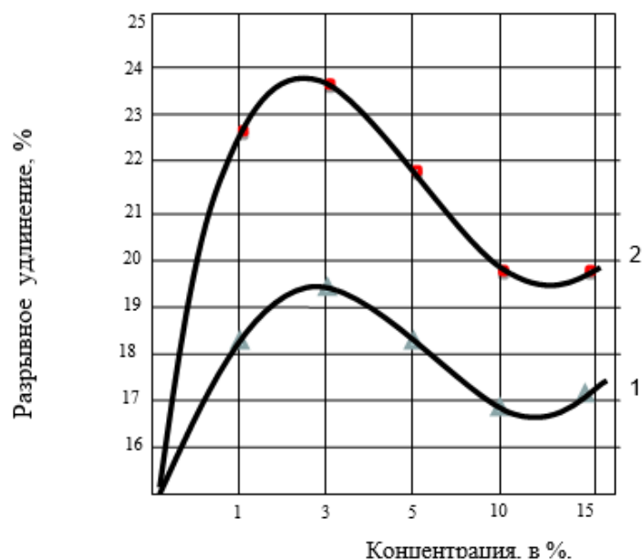
Рис. 3. Показатели разрывного удлинения (%), хлопчатобумажных тканей, обработанных модифицированным мочевино-формальдегидным олигомером: по основе - (1) и утку - (2)
