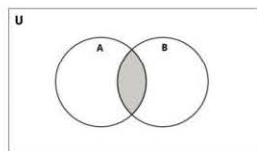
Рис. 13. Диаграмма «Пересечение»
