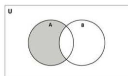
Рис. 14. Диаграмма «Разность»
