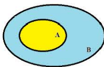
Рис. 10. Диаграмма «Подмножество»
