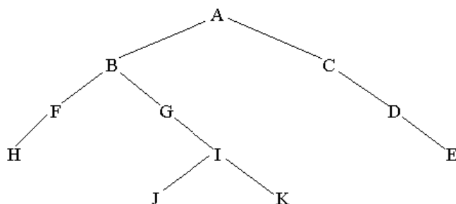
Рис. 29. Бинарное дерево
