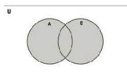
Рис. 12. Диаграмма «Объединение»
