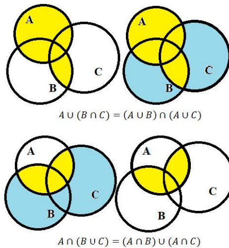
Рис. 16. Операция «Дистрибутивность»
